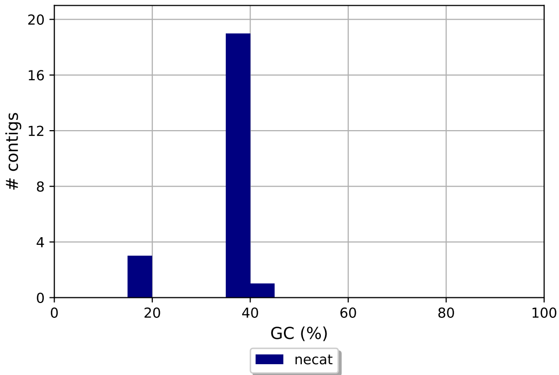
necat GC content
