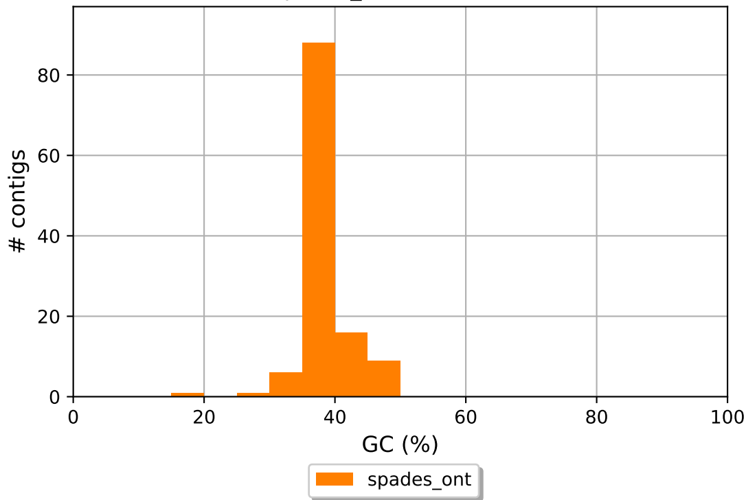
spades_ont GC content
