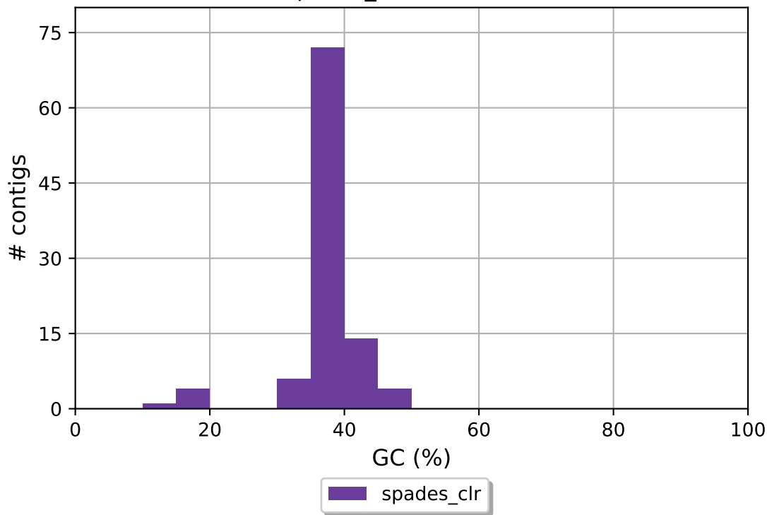
spades_clr GC content
