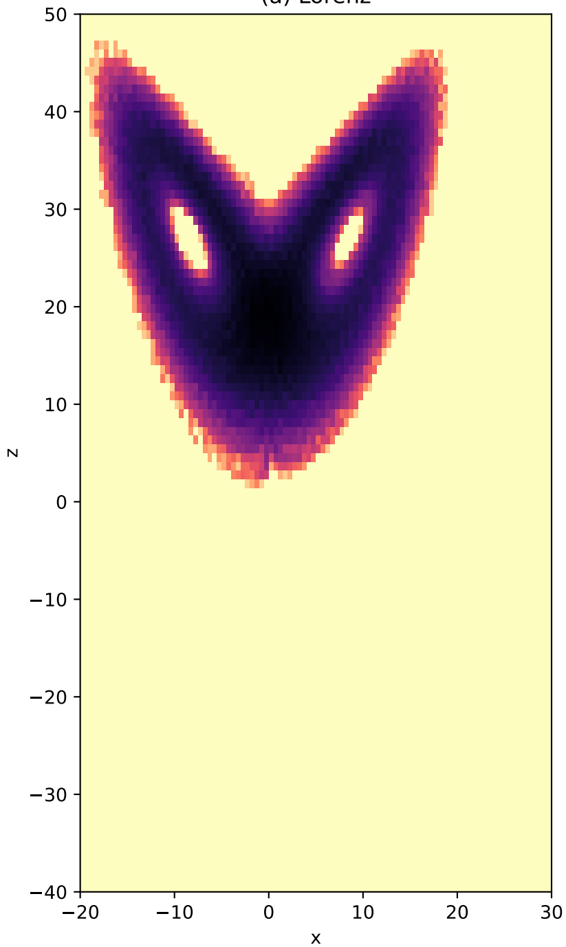
(a) Lorenz
