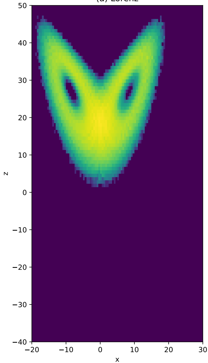
(a) Lorenz
