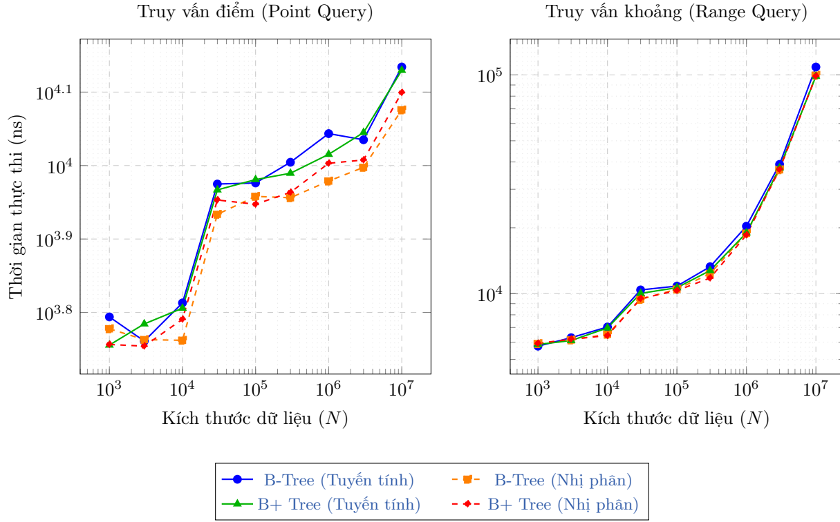
Hình 1 So sánh hiệu năng truy vấn điểm và truy vấn khoảng theo kích thước dữ liệu ( N ).
