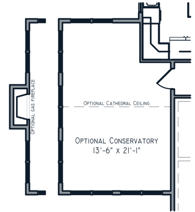
OPTIONAL CONSERVATORY
