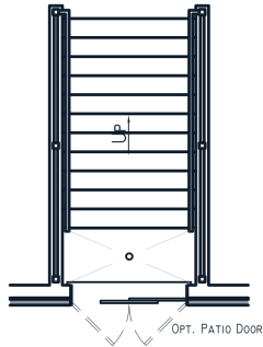
OPTIONAL 7' AREAWAY
