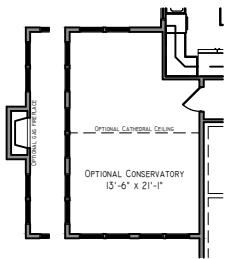
Optional Conservatory
