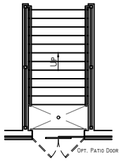
Optional 7' Areaway
