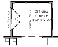
Optional Sunroom
