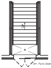
Optional 7' Areaway
