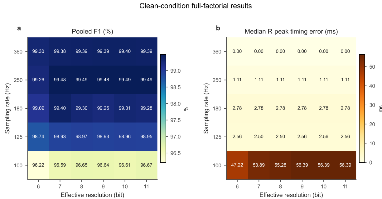
图4 干净条件下30种配置的F1、时间误差与资源指标热力图。
