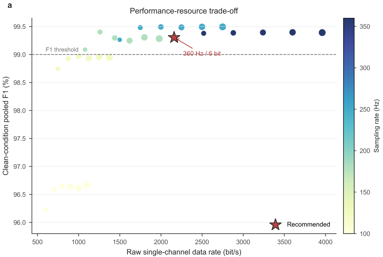
图8 干净条件性能与原始数据率的帕累托权衡。
