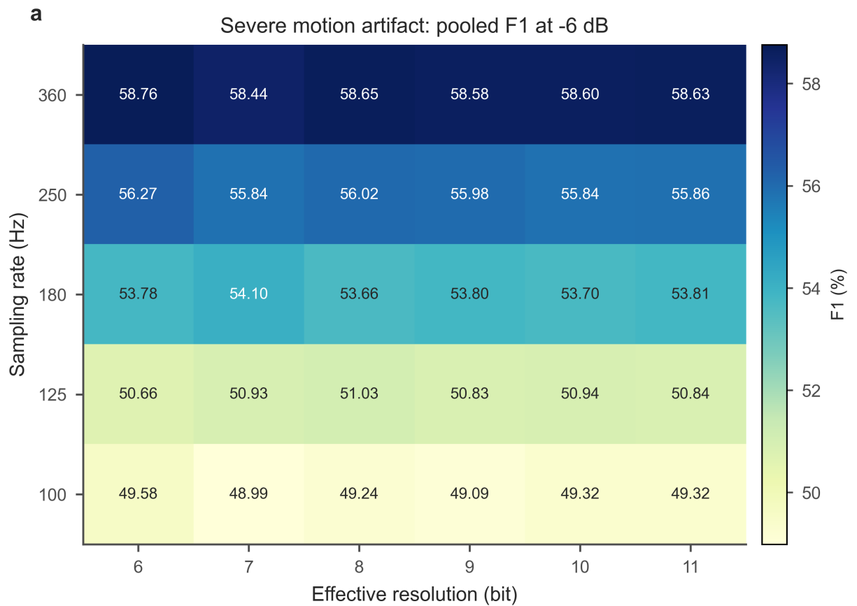
图7 严重运动伪影下的全因子性能热力图。
