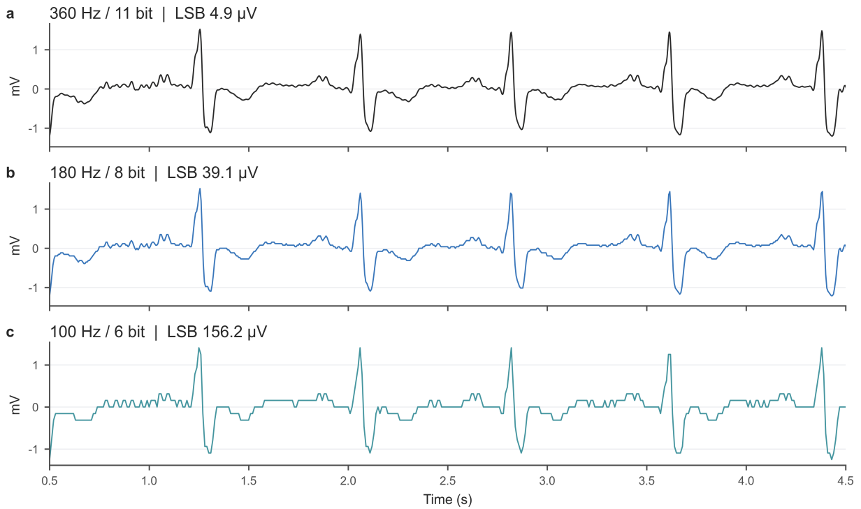
图3 不同虚拟采集配置的代表性ECG波形。
