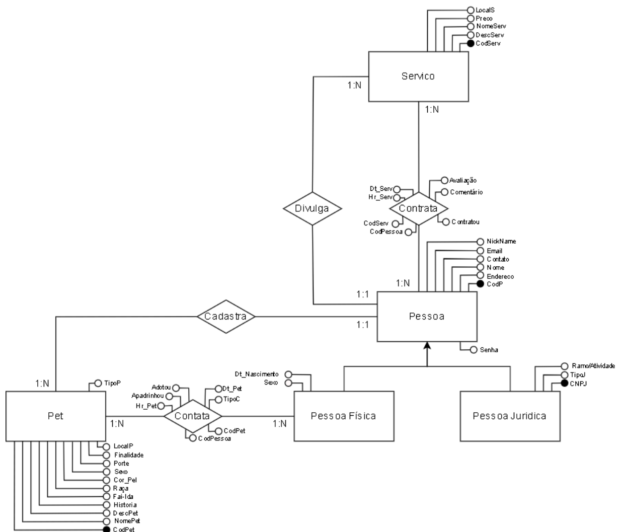
Figura 5: Diagrama de Entidade e Relacionamento
