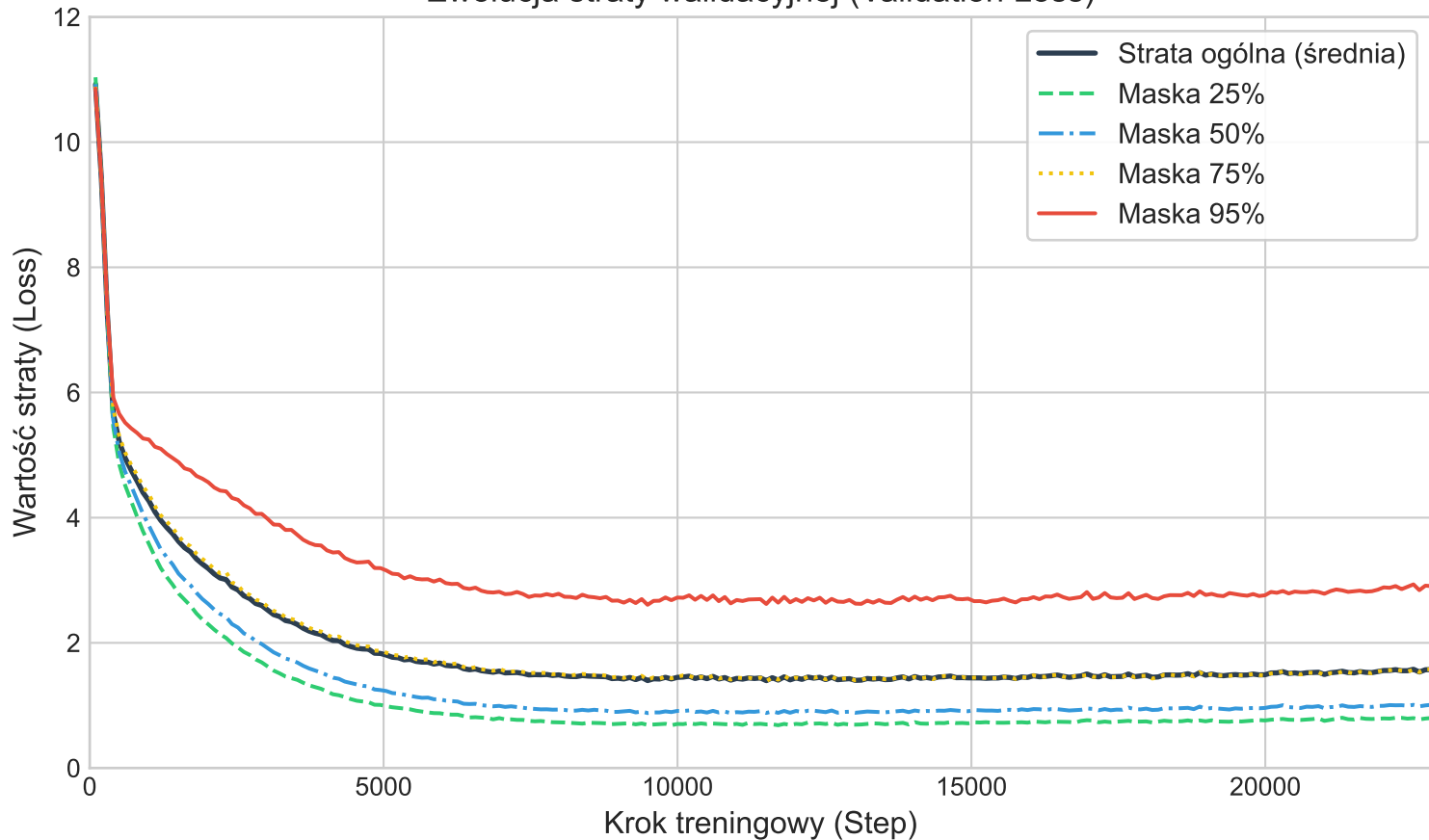
Ewolucja straty walidacyjnej (Validation Loss)
