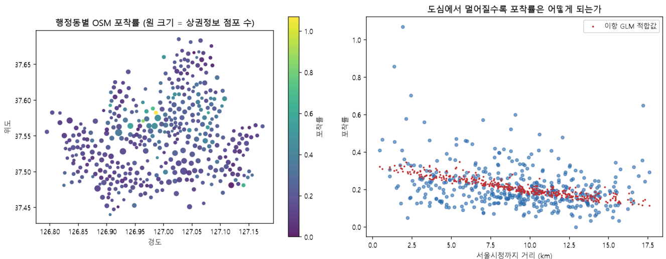
그림 3.4 왼쪽은 행정동 중심점에 찍은 OSM 포착률이며 밝을수록 높고 원 크기는 상가정보 점포 수 — 시청과 종로·중구 일대가 밝고 외곽으로 갈수록 어두워짐. 오른쪽은 서울시청까지 거리에 따른 포착률과 회귀 적합값으로, 거리가 늘수록 적합값이 0.30에서 0.12 부근까지 내려감. 같은 거리에서도 점이 위아래로 크게 흩어지는데, 거리만으로 설명되지 않는 동별 차이가 그만큼 크다는 뜻임
