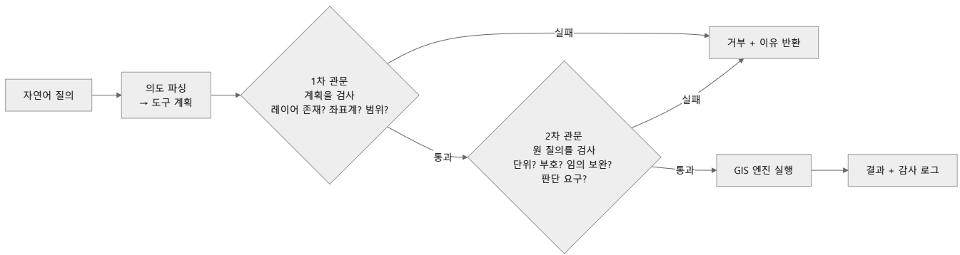
그림 7.1 질의 처리 순환과 두 층의 검증 관문. 1차 관문은 모델이 만든 계획을 검사하고, 2차 관문은 원 질의를 함께 본다. 계획으로 환원되지 않는 정보(단위·부호·요청의 성격)는 2차 관문에서만 잡힌다.
