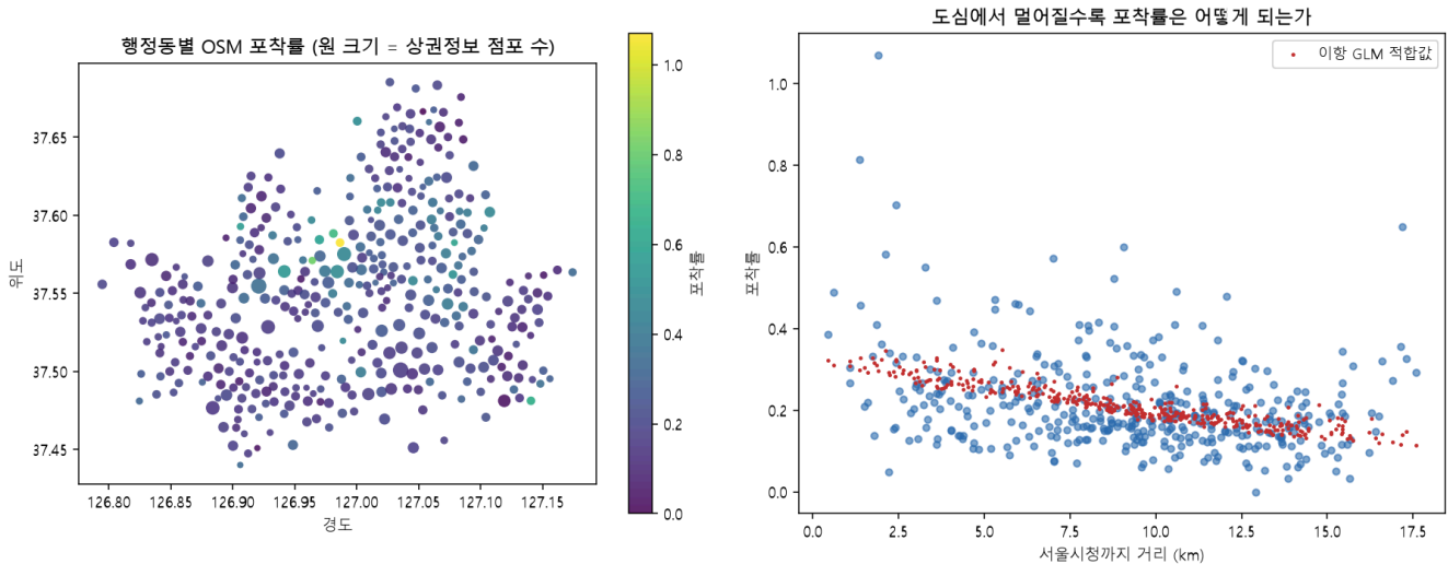
그림 3.4 왼쪽은 행정동 중심점에 찍은 OSM 포착률이며 밝을수록 높고 원 크기는 상가정보 점포 수 — 시청과 종로·중구 일대가 밝고 외곽으로 갈수록 어두워짐. 오른쪽은 서울시청까지 거리에 따른 포착률과 이항 GLM 적합값으로, 거리가 늘수록 적합값이 0.30에서 0.12 부근까지 내려감. 같은 거리에서도 점이 위아래로 크게 흩어지는데, 이 흩어짐이 위의 과대산포와 잔차 공간 자기상관에 해당함
