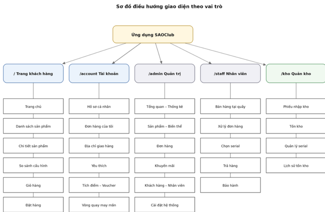
Hình 50: Sơ đồ điều hướng giao diện
