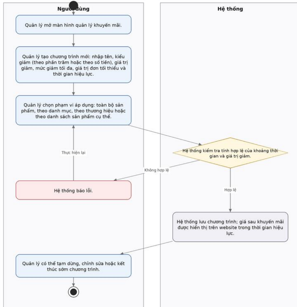
Hình 34: Activity Diagram quản lý khuyến mãi và phiếu giảm giá
