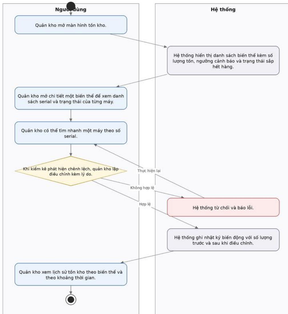
Hình 29: Activity Diagram quản lý tồn kho và số serial
