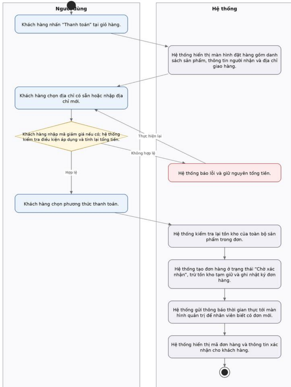
Hình 11: Activity Diagram đặt hàng trực tuyến
