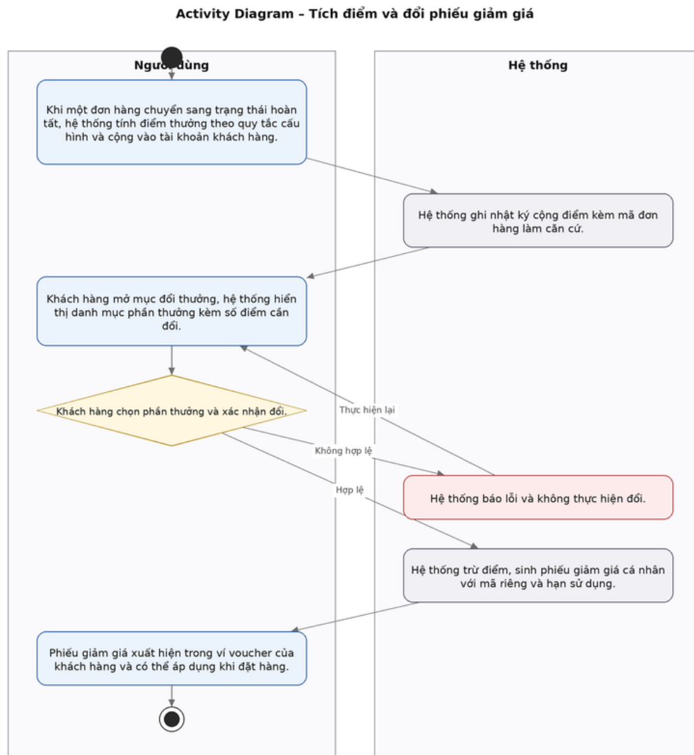
Hình 16: Activity Diagram tích điểm và đổi phiếu giảm giá
