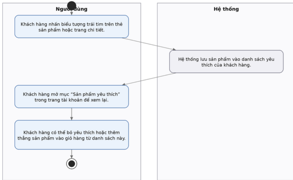
Hình 15: Activity Diagram quản lý sản phẩm yêu thích
