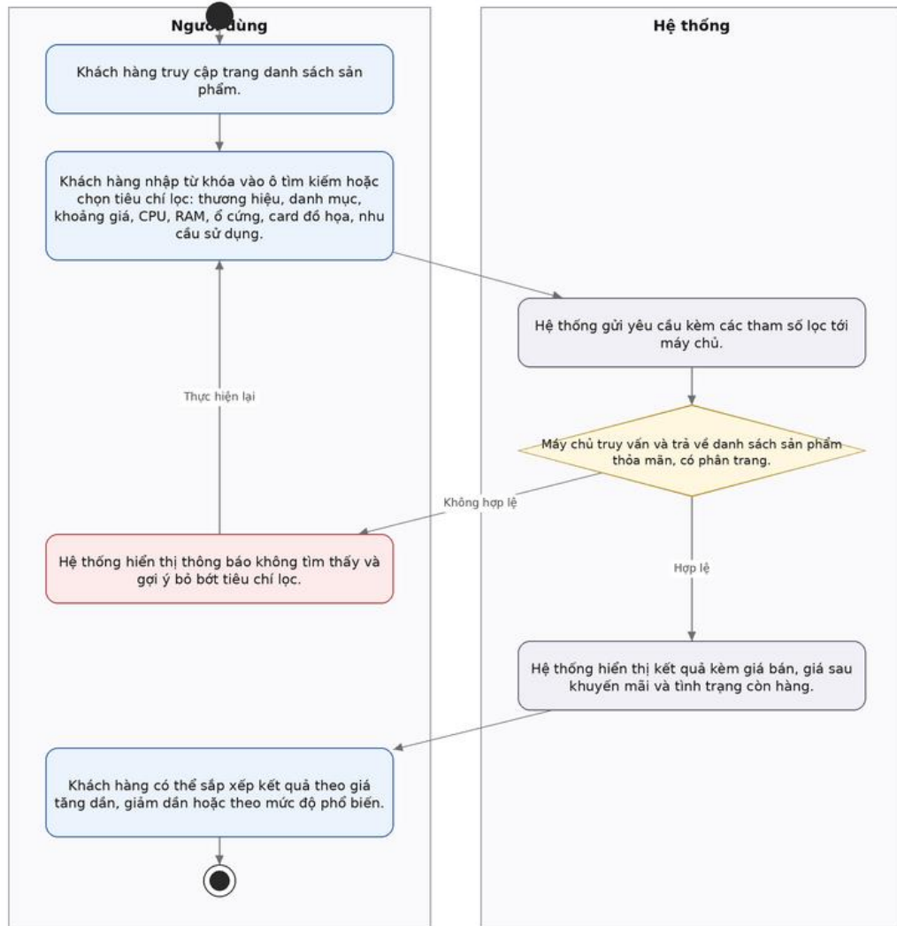
Hình 8: Activity Diagram tìm kiếm và lọc sản phẩm
