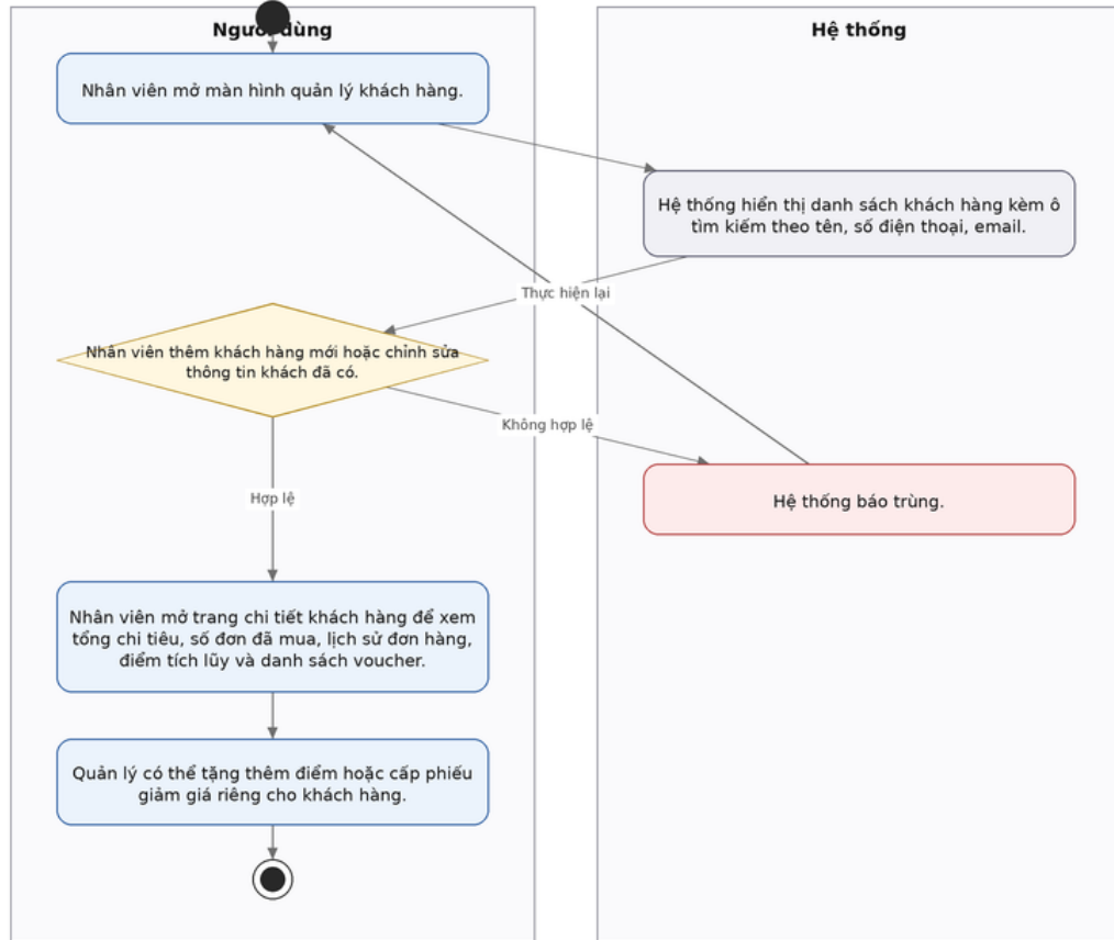
Hình 36: Activity Diagram quản lý khách hàng
