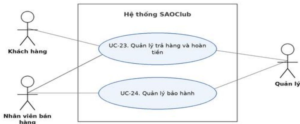
Hình 30: Use Case nhóm trả hàng và bảo hành
