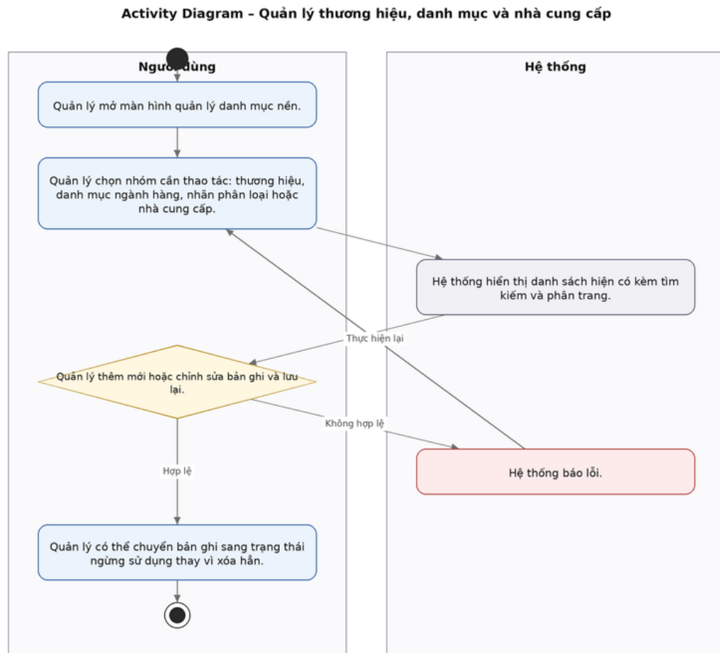
Hình 26: Activity Diagram quản lý thương hiệu, danh mục và nhà cung cấp
