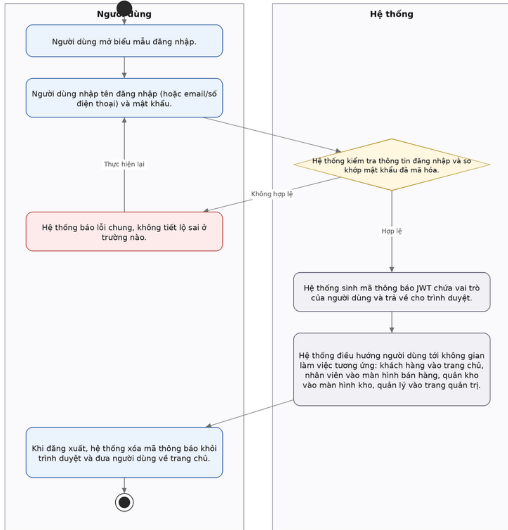
Hình 5: Activity Diagram đăng nhập và đăng xuất
