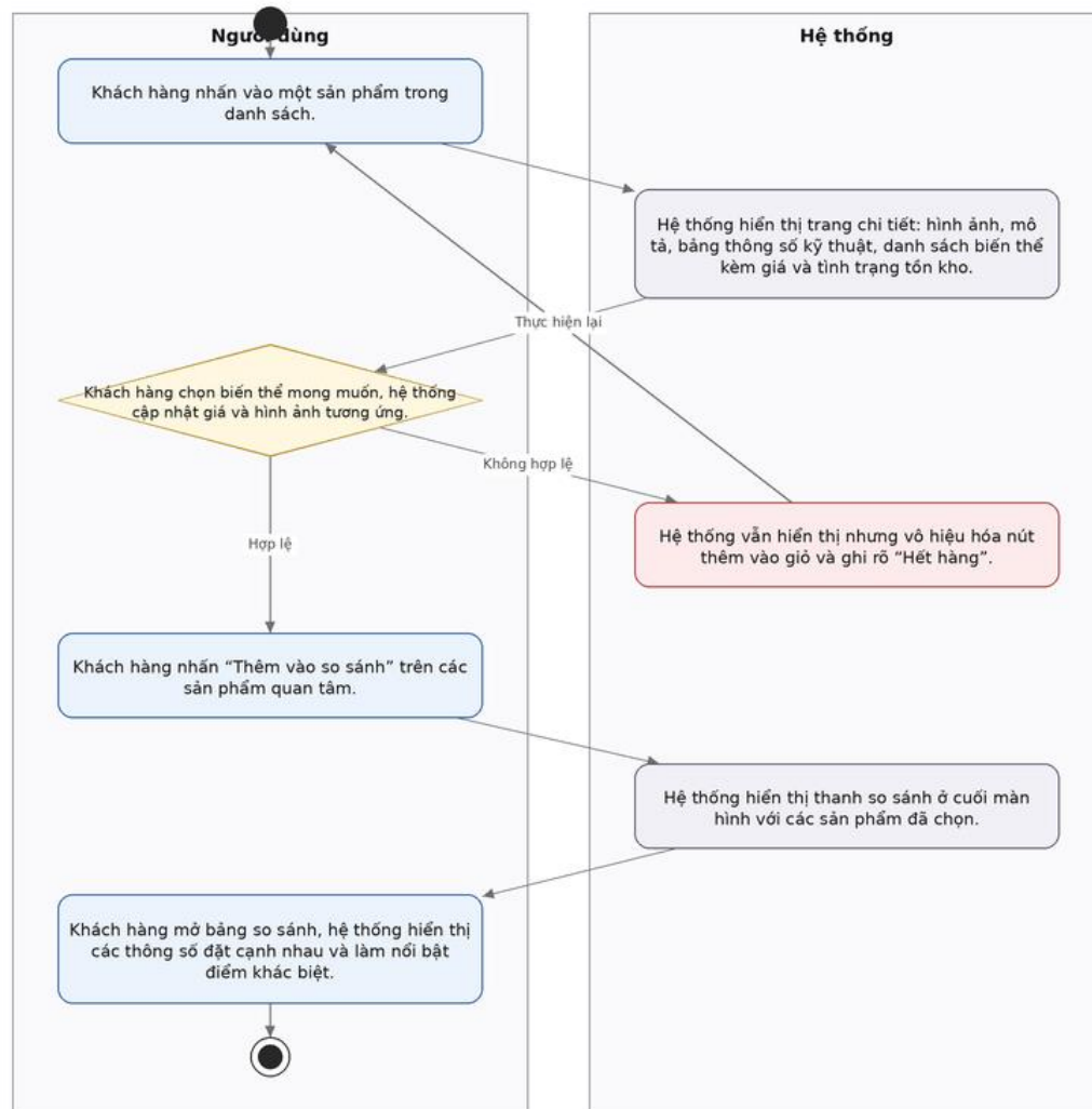
Hình 9: Activity Diagram xem chi tiết và so sánh biến thể sản phẩm
