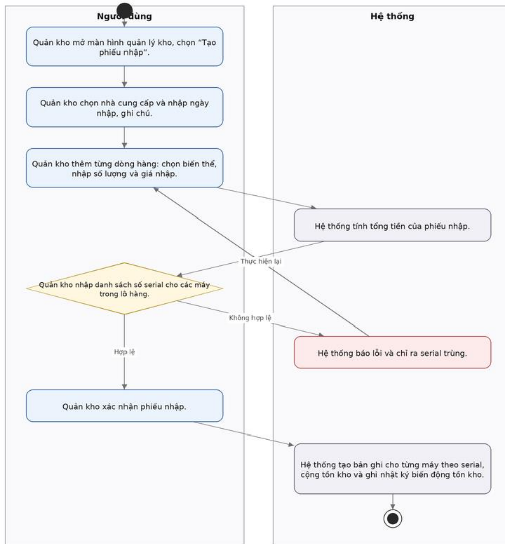
Hình 28: Activity Diagram quản lý phiếu nhập kho
