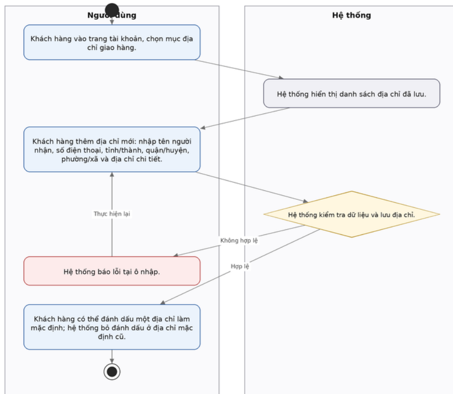
Hình 12: Activity Diagram quản lý địa chỉ giao hàng
