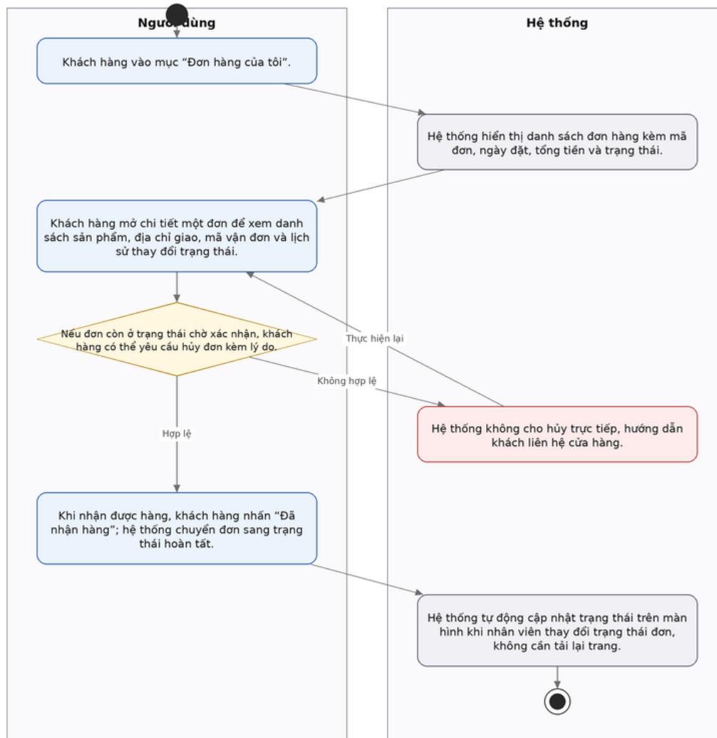
Hình 13: Activity Diagram theo dõi và quản lý đơn hàng của khách hàng
