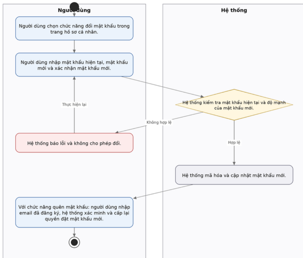
Hình 6: Activity Diagram đổi mật khẩu và quên mật khẩu
