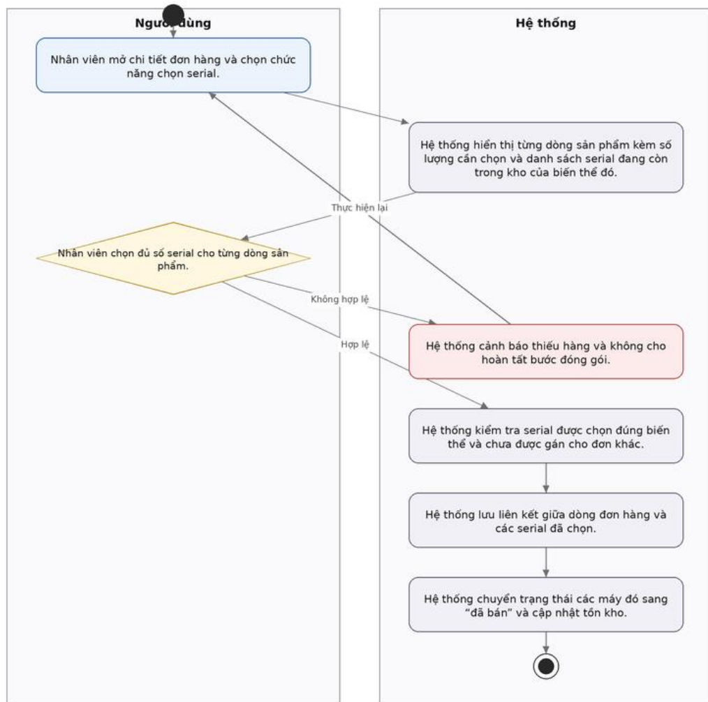
Hình 21: Activity Diagram chọn serial và đóng gói đơn hàng
