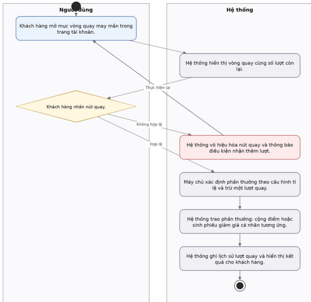
Hình 17: Activity Diagram tham gia vòng quay may mắn
