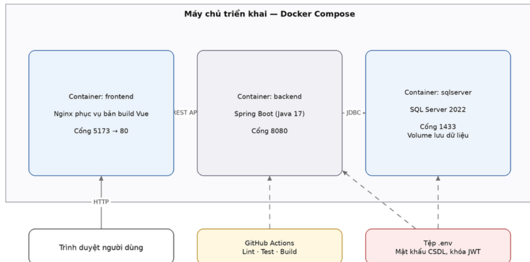
Hình 76: Sơ đồ triển khai hệ thống
