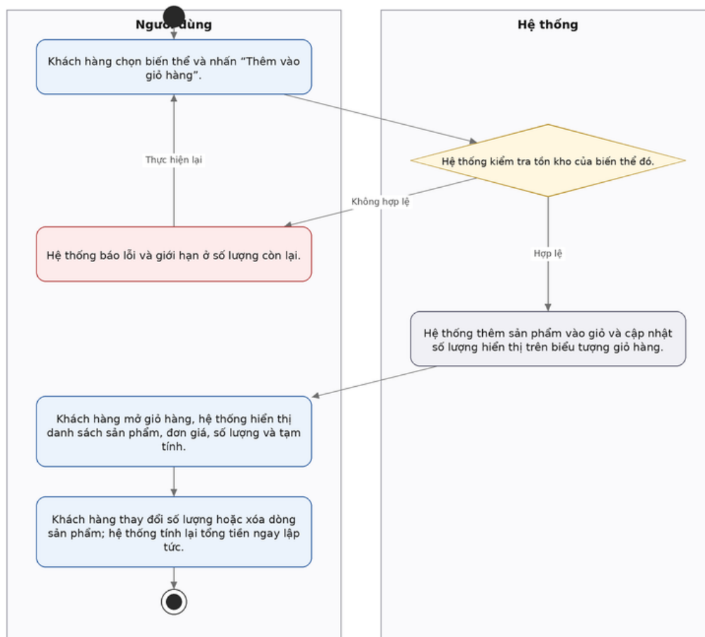
Hình 10: Activity Diagram quản lý giỏ hàng
