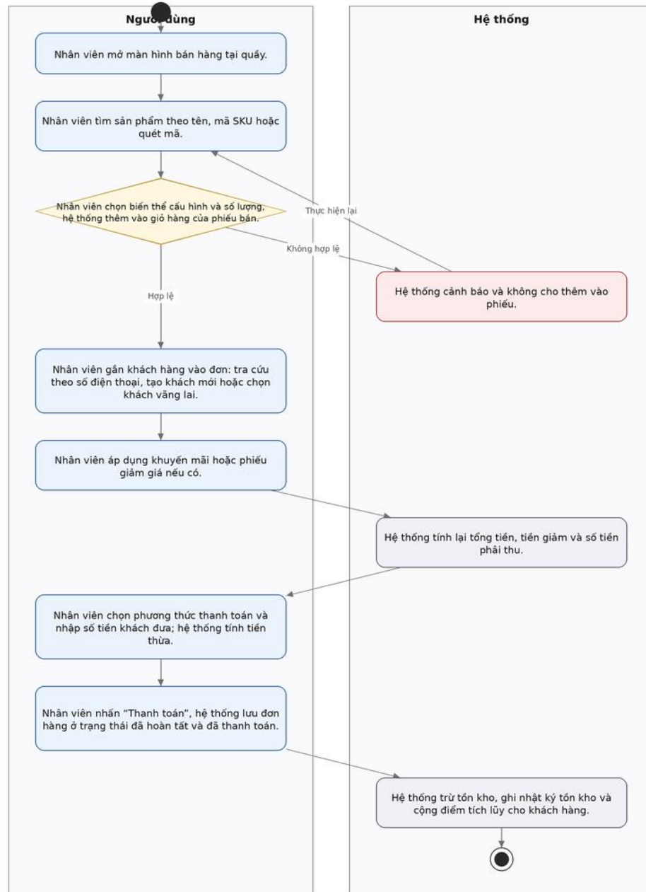
Hình 19: Activity Diagram bán hàng tại quầy
