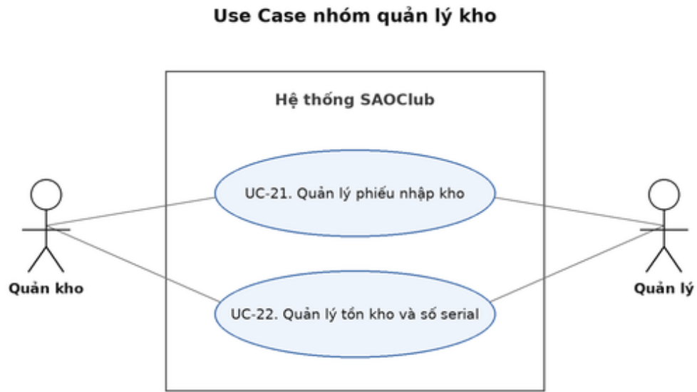
Hình 27: Use Case nhóm quản lý kho
