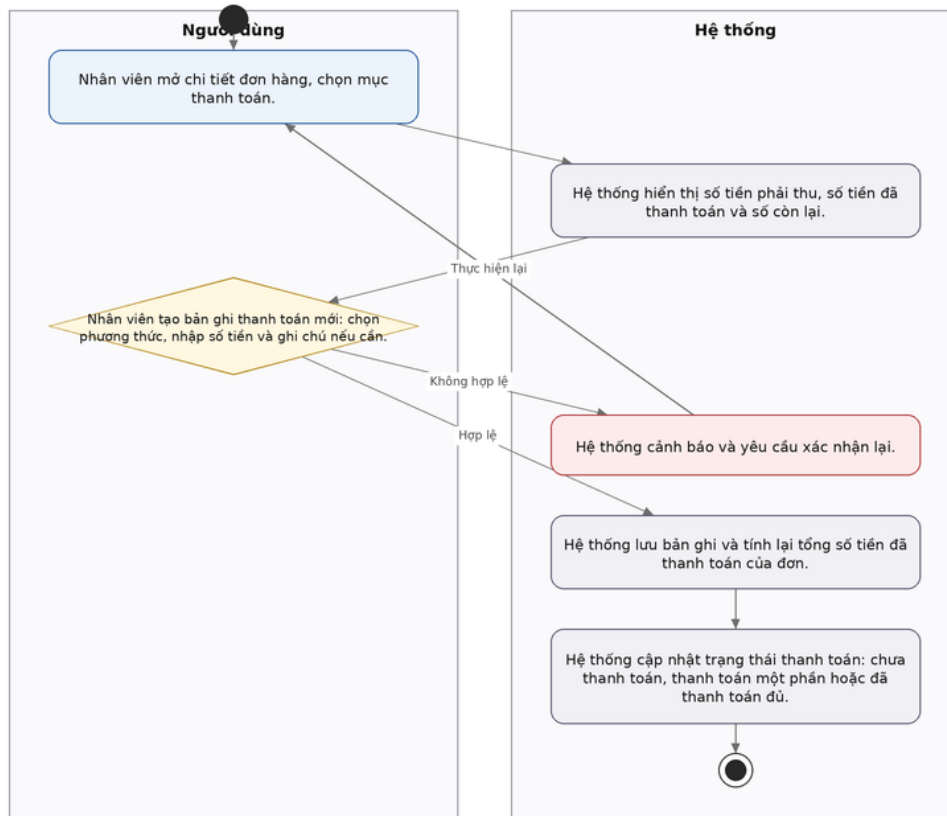
Hình 22: Activity Diagram quản lý thanh toán
