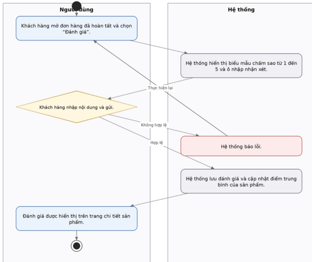
Hình 14: Activity Diagram đánh giá sản phẩm
