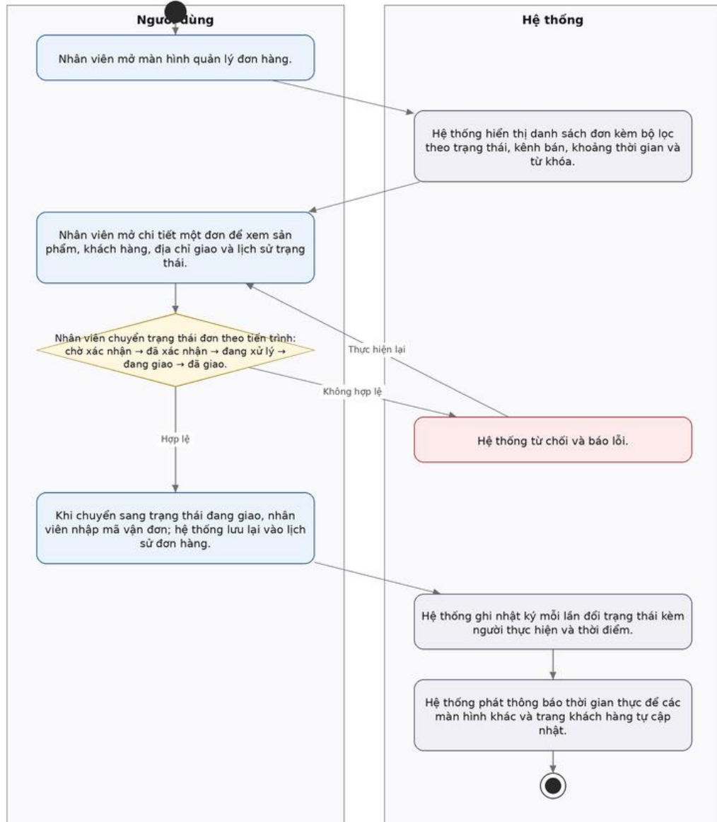
Hình 20: Activity Diagram quản lý đơn hàng
