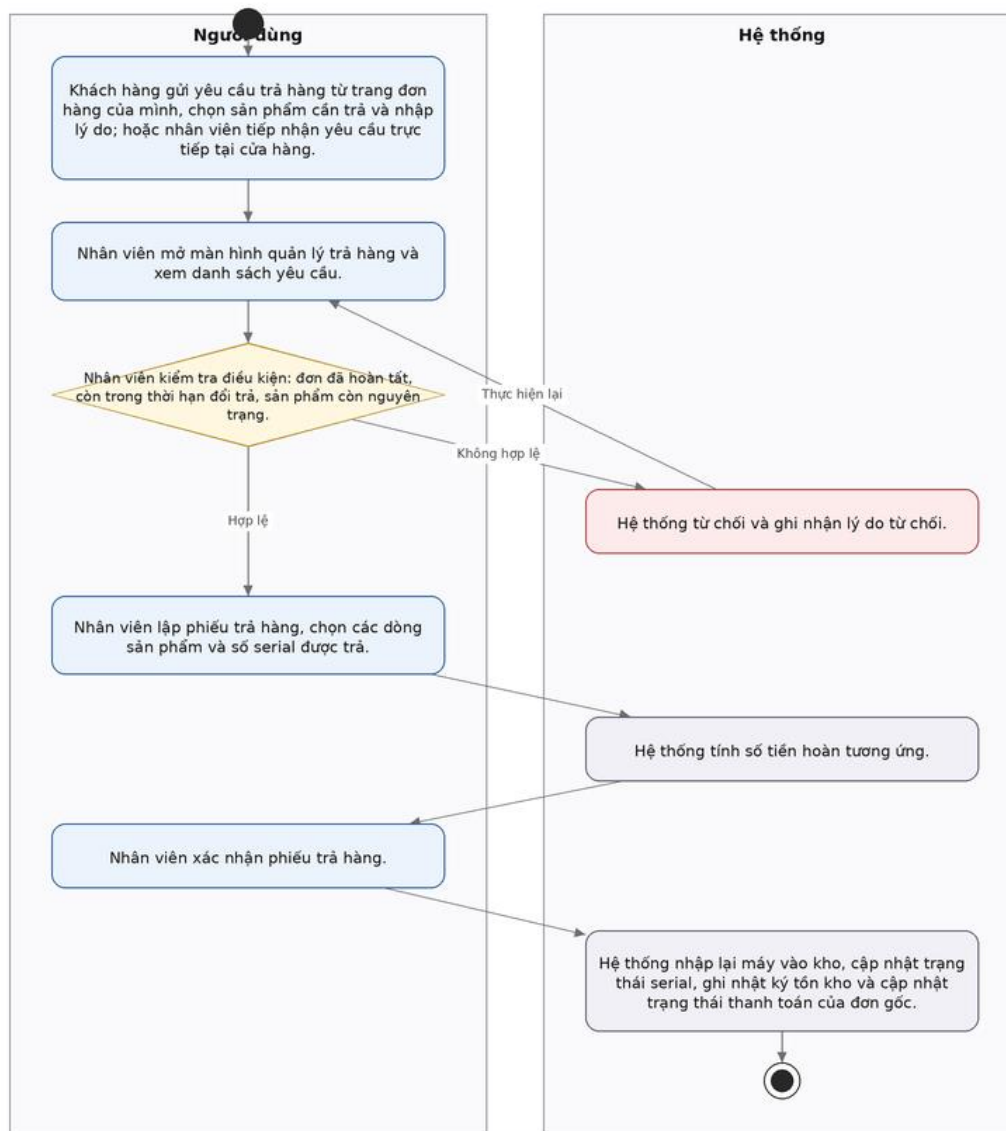
Hình 31: Activity Diagram quản lý trả hàng và hoàn tiền
