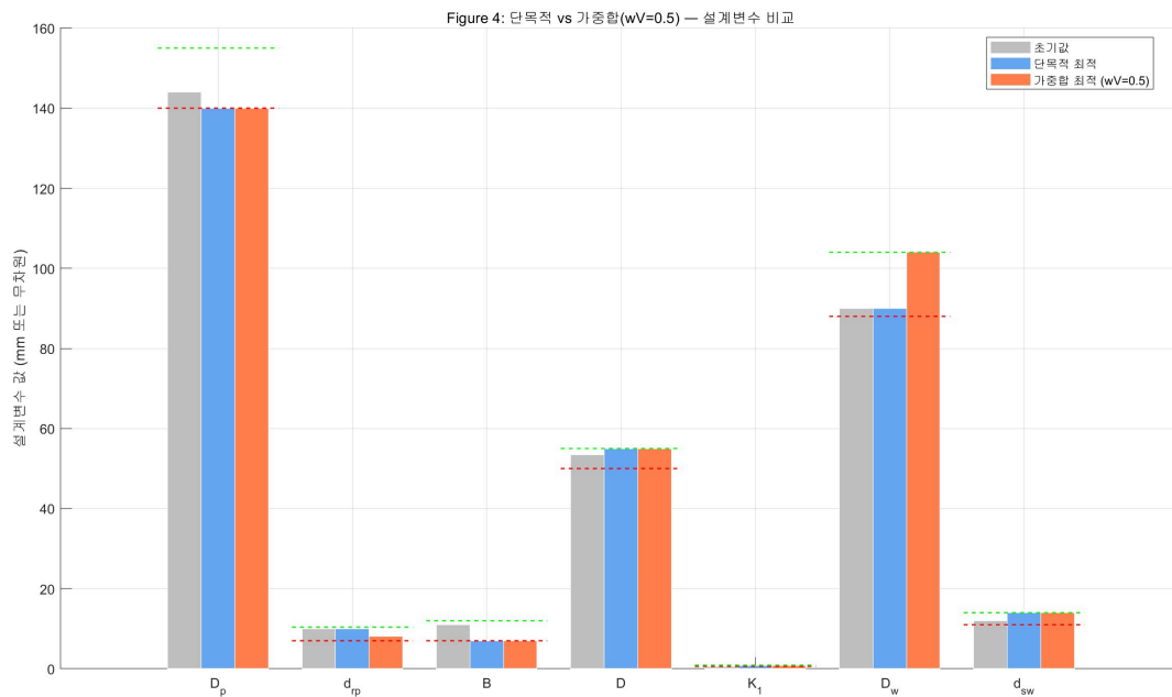
[Figure 4: 단목적 vs 가중합( wV=0.5 ) 설계변수 비교 — 초기값 대비 최적값 (단목적: 파란색, 가중합: 주황색)]
