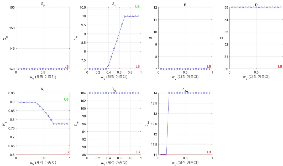
가중치 w_V 에 따른 최적 설계변수 변화
