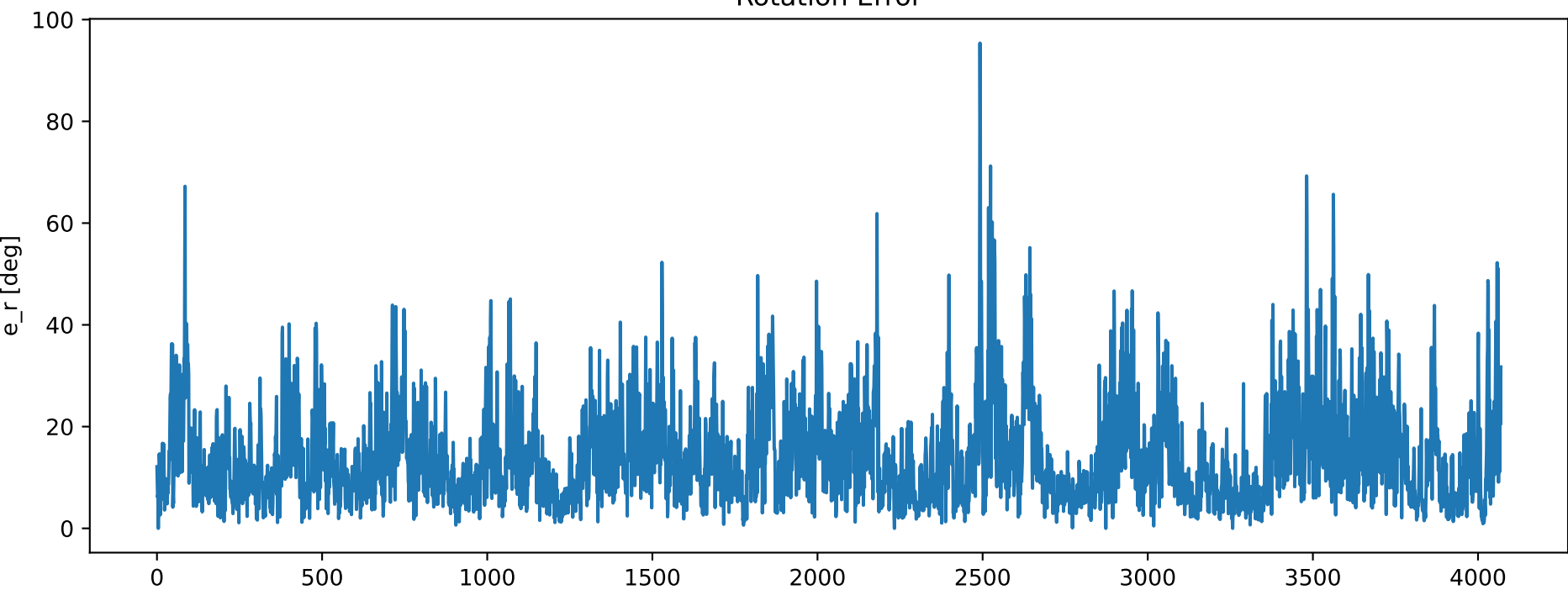
Rotation Error
