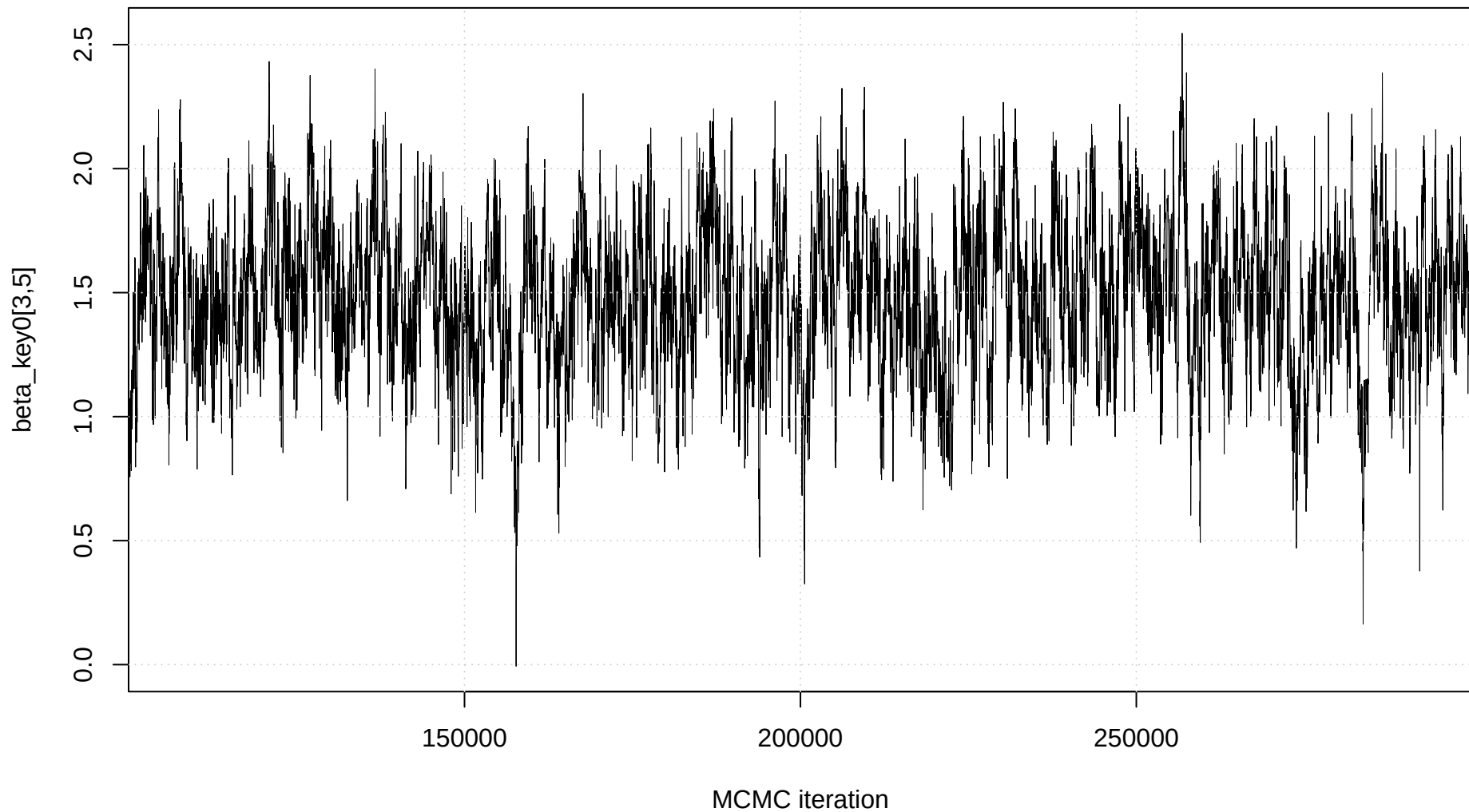
Trace plot: beta_key0[3,5]
