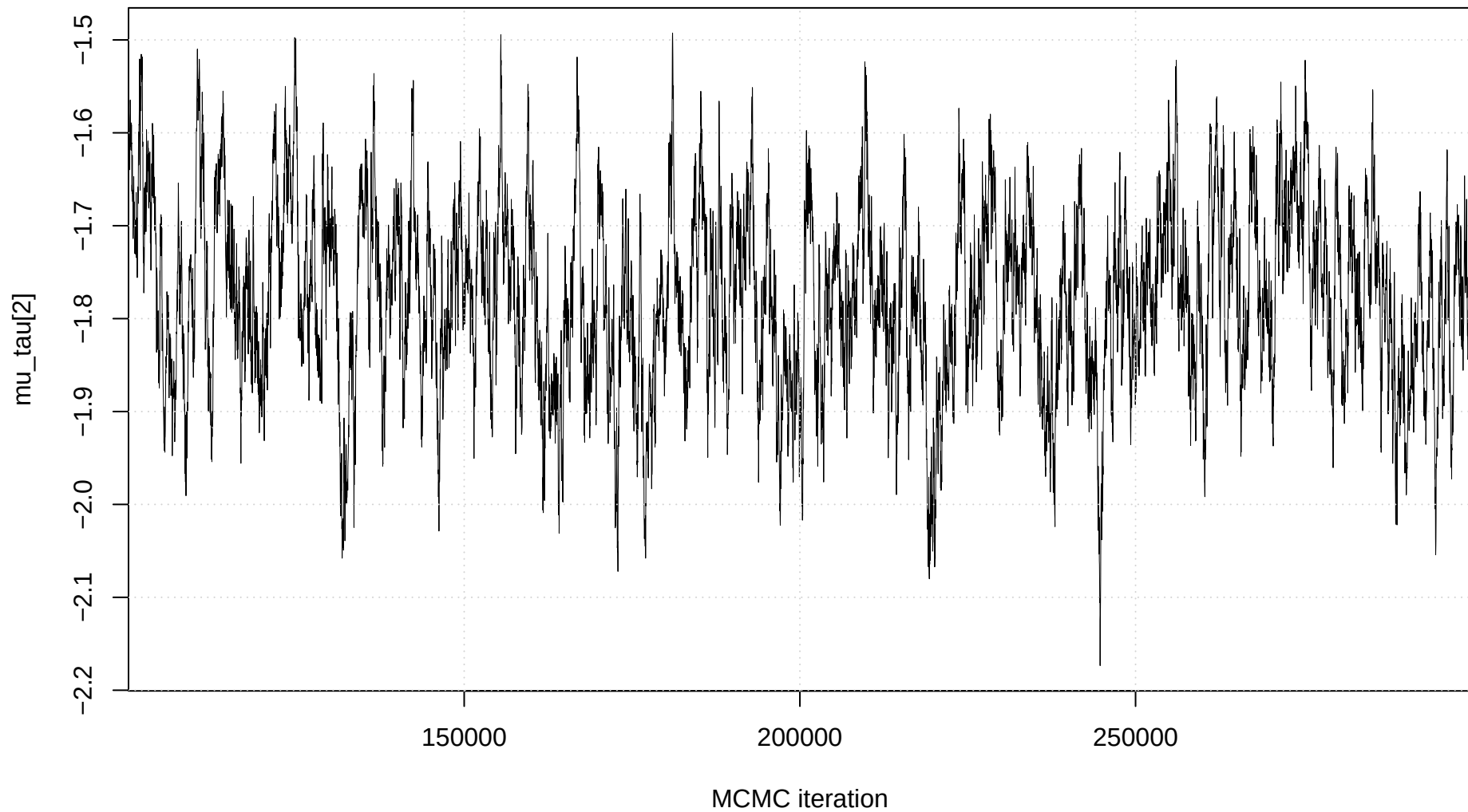
Trace plot: mu_tau[2]
