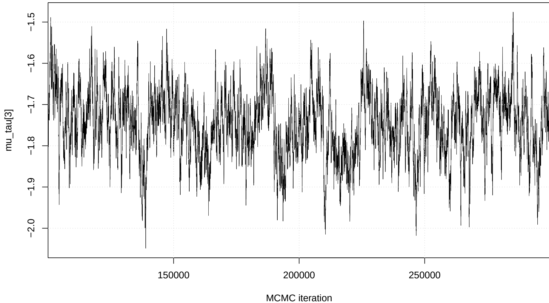
Trace plot: mu_tau[3]
