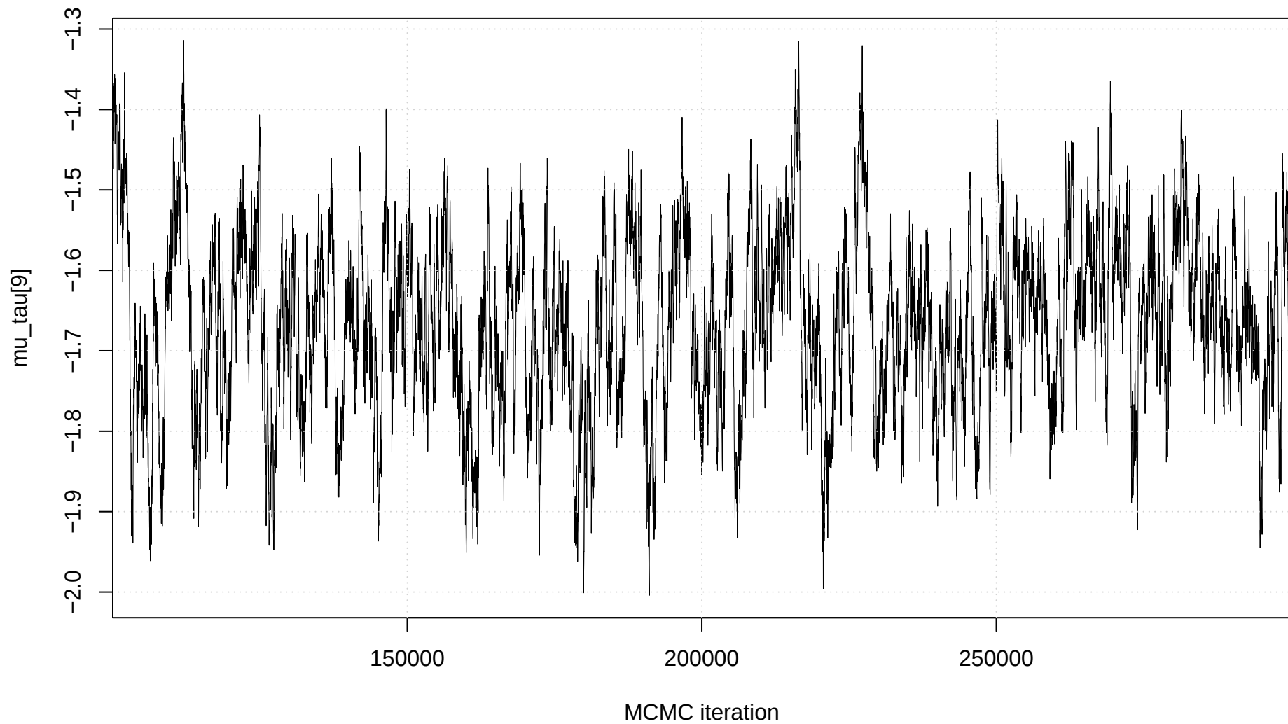
Trace plot: mu_tau[9]
