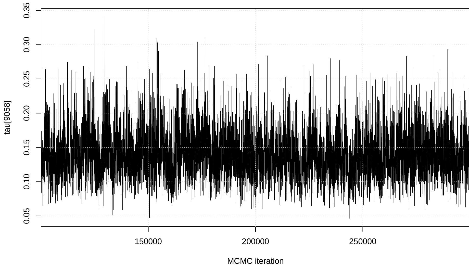
Trace plot: tau[9058]
