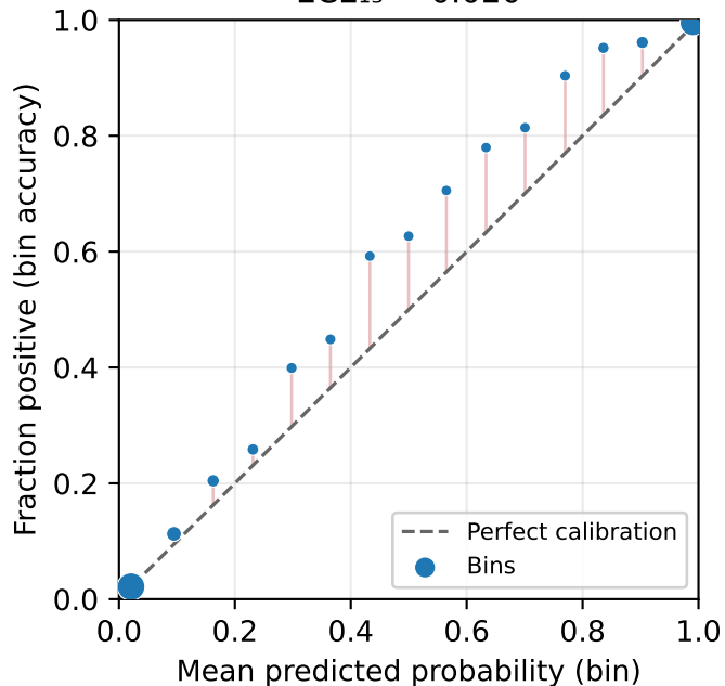
C1: PCam \rightarrow PCam test ECE_{15} = 0.020
