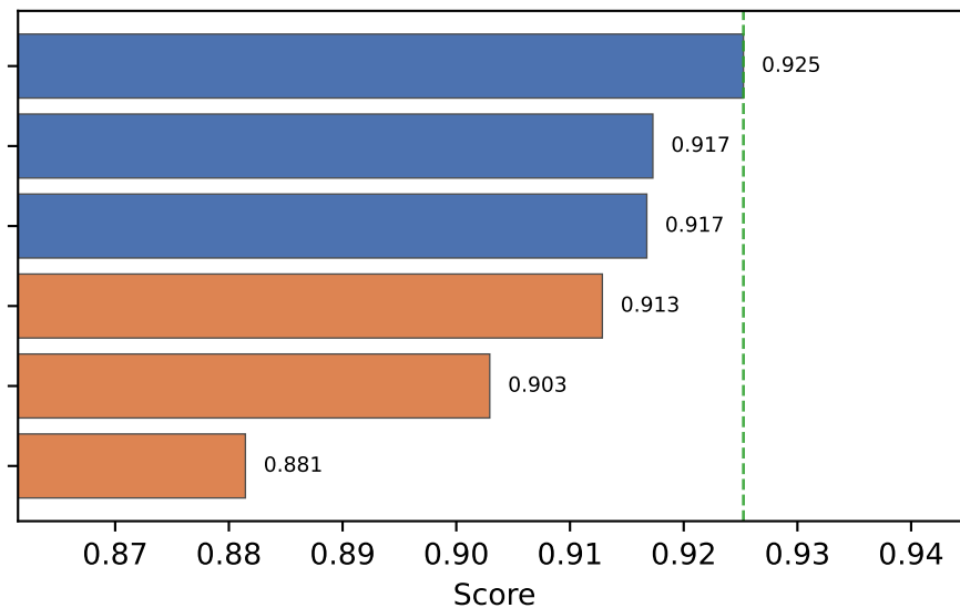
Test F1 @ 0.5
