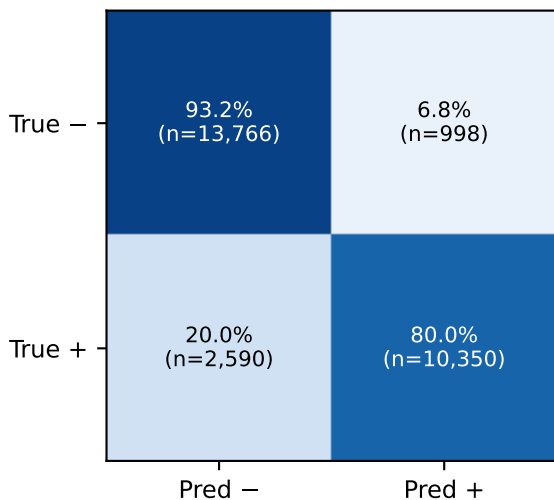
PCam → PCam
