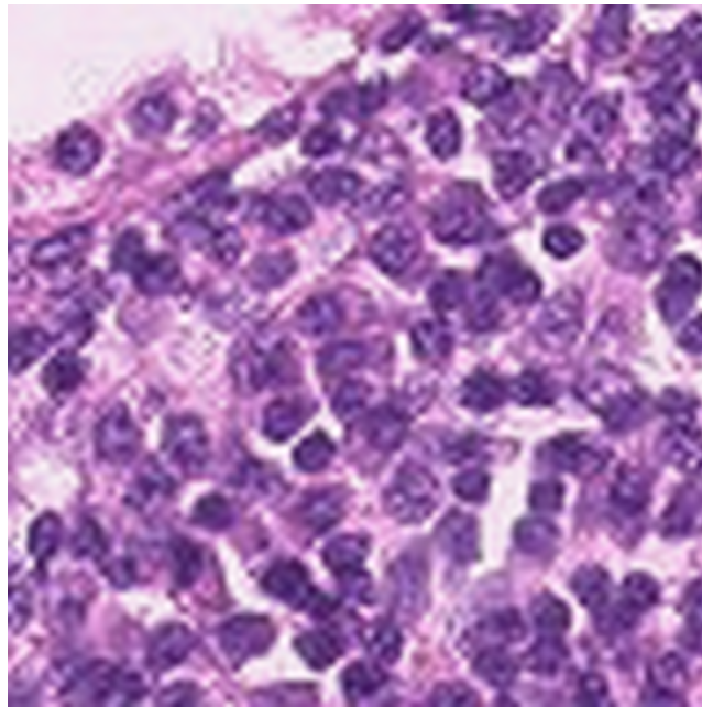
Reinhard
