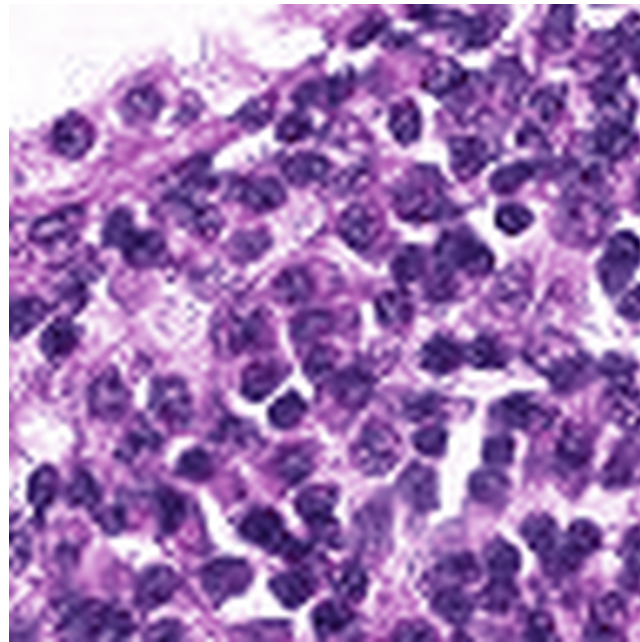
Vahadane
