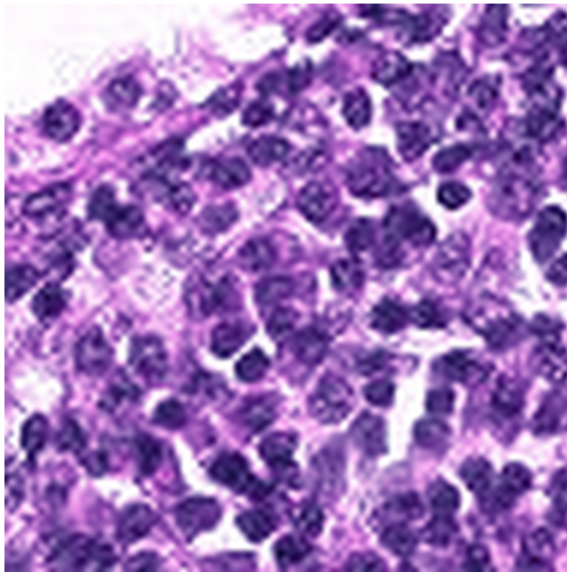
Macenko
