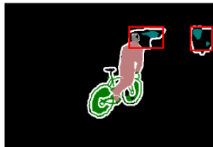
Argmax-prob
