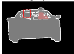
Argmax-prob
