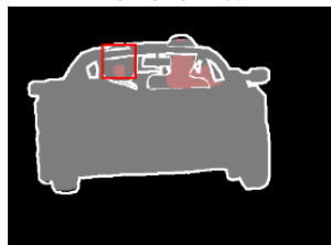
RankSEG-RMA
