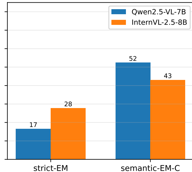
non-Latin (ar/ja/kr/ru/th)
