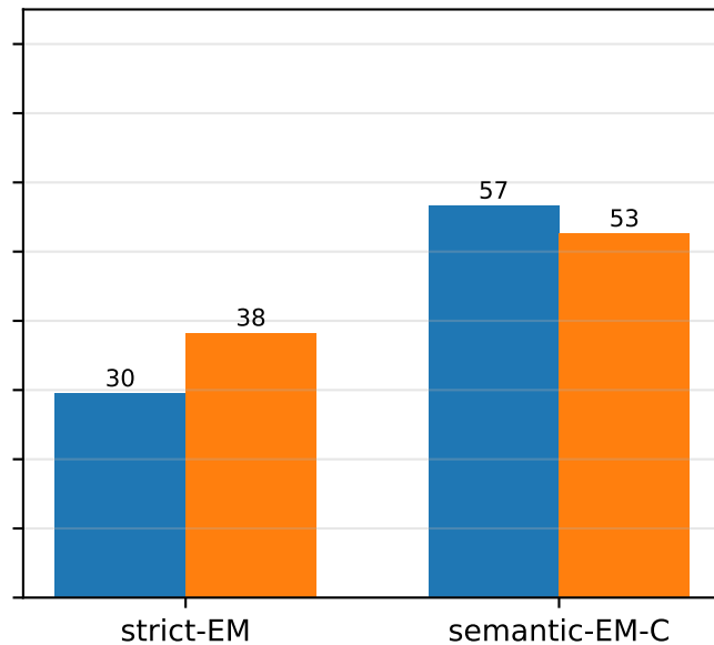
Latin (de/fr/it/vi)
