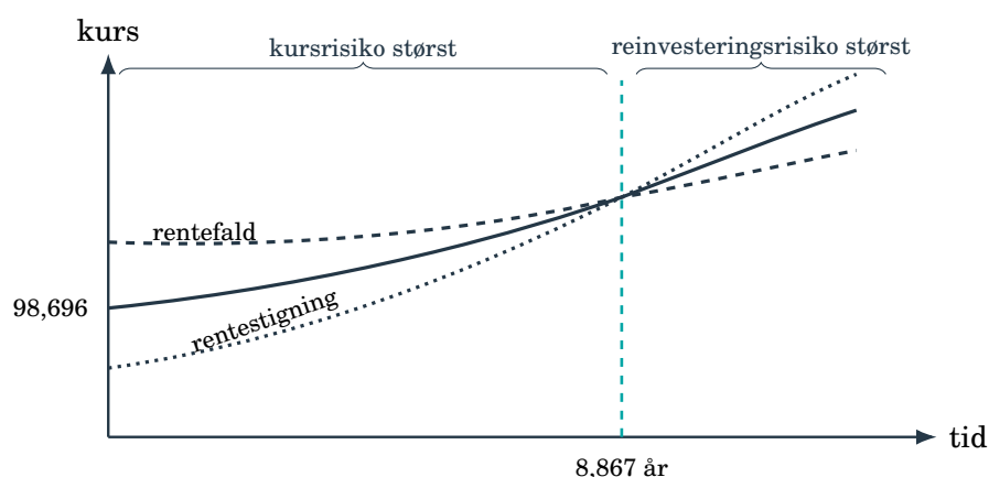
Figur 4.4: Immuniseringshorisonten. Ved varighedshorisonten opvejer kursrisiko og reinvesteringsrisiko hinanden under simple antagelser.
