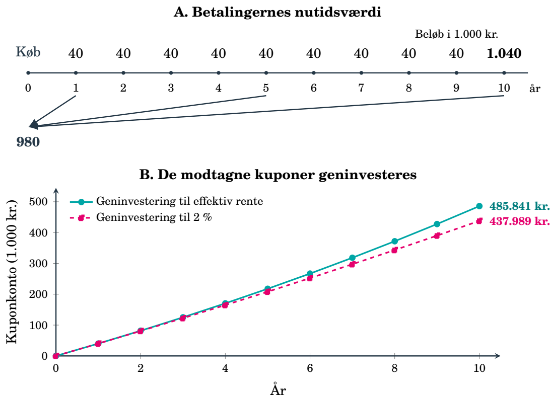
Figur 2.8: Den samme obligations betalinger bruges til to beregninger. I A viser pilene diskontering af udvalgte betalinger tilbage til købet. I B viser punkterne kuponkontoen lige efter hver årlig betaling ved to geninvesteringsrenter. Hovedstolen indgår først i slutformuen ved udløb.
