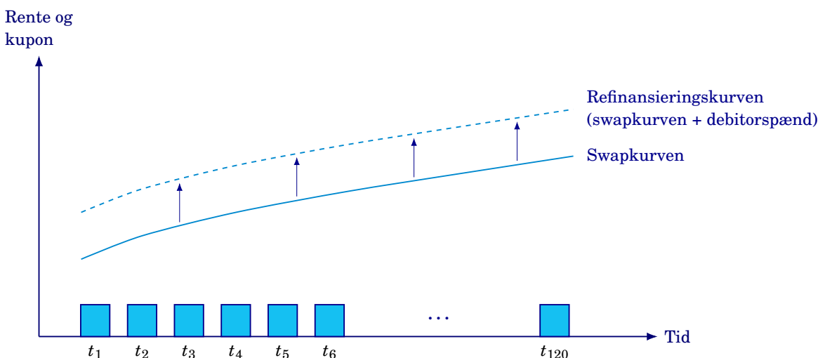
Figur 6.7: Betalingsterminerne og låntagers refinansieringskurve, som her fremkommer ved at lægge debitorspændet til swapkurven. De lige høje søjler viser skematisk en annuitet uden førtidig indfrielse. Når betalingerne vurderes med den højere refinansieringskurve, diskonteres de hårdere. Kurvernes form er skematisk; det lodrette spænd er pointen. Egen illustration.
