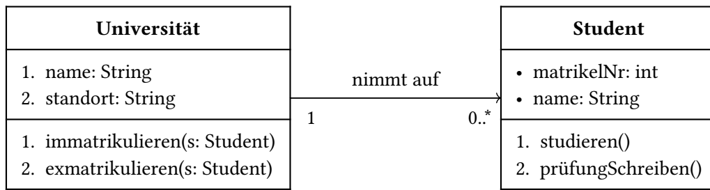
Abbildung 1: Robustes UML-Klassendiagramm auf Basis von Typst-Grids.
