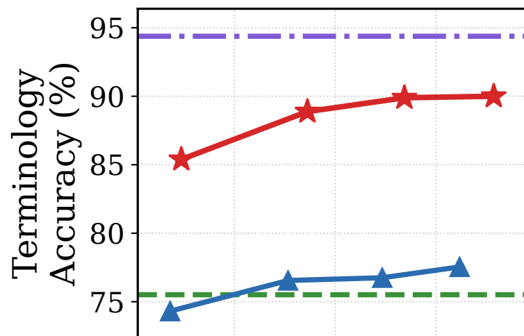
En-Zh
