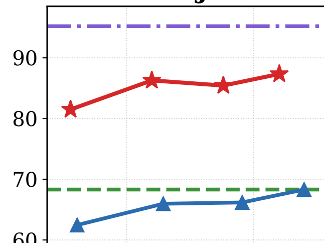
En-Ja
