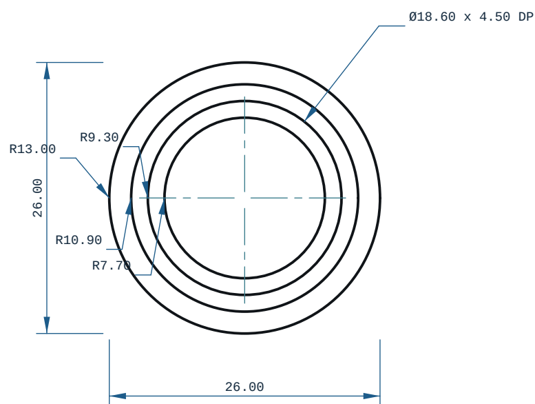
TOP VIEW X ? Y ?
