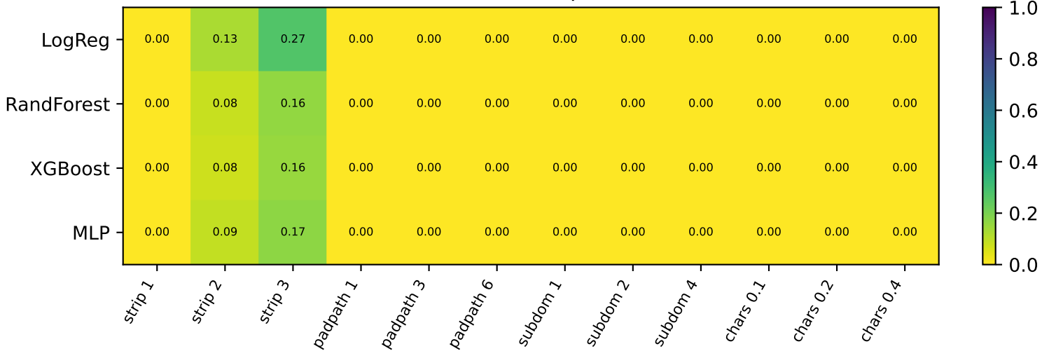
False-positive rate (benign flagged)
