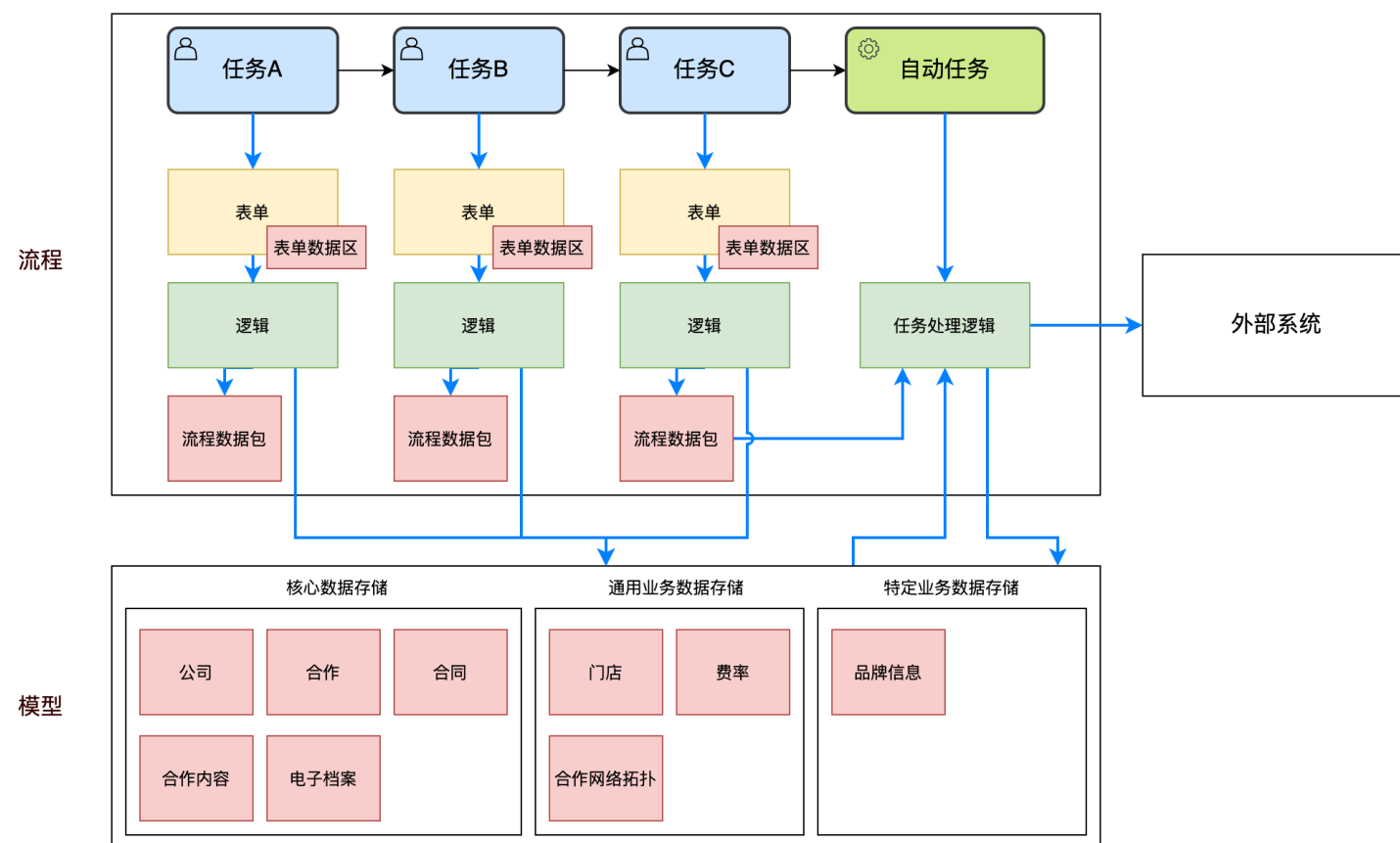
流程-模型数据流向示例
