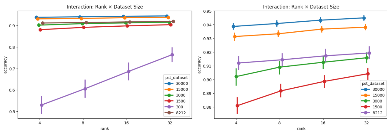
Рисунок Влияние ранга на качество модели.
