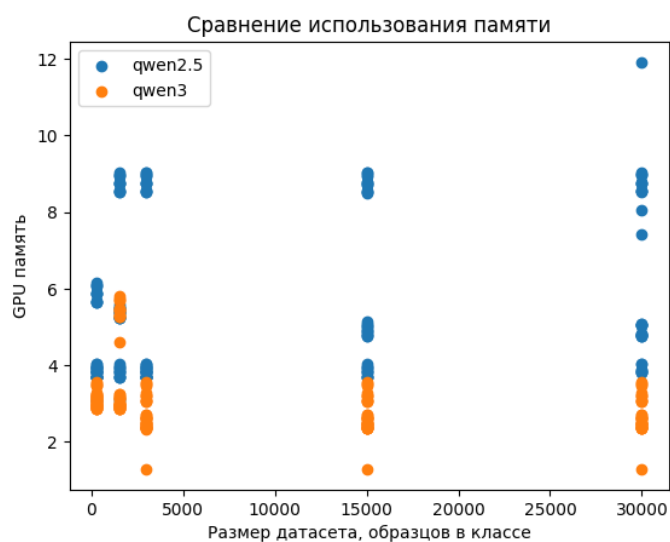
Рисунок 8. Сравнение использования памяти
