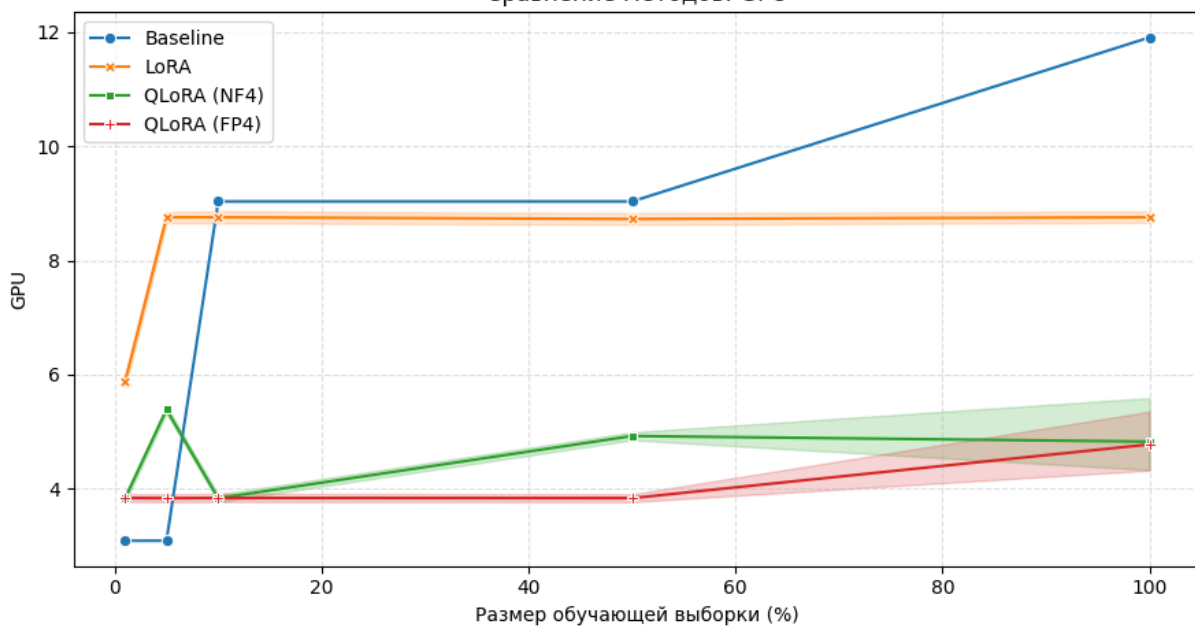
Сравнение методов: GPU
