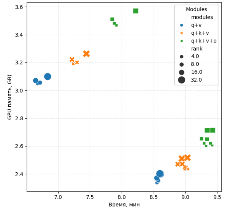
Точечная диаграмма расположения различных конфигураций настроек относительно затратам памяти и времени обучения для Qwen3-0.6B (EN)
