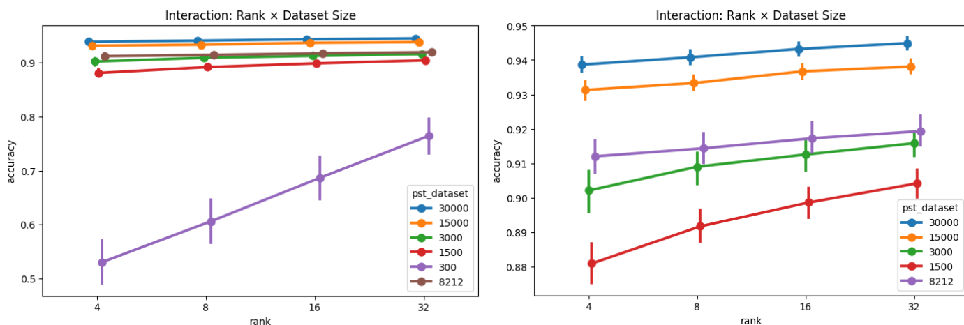
Рисунок 7. Влияние ранга на качество модели.
