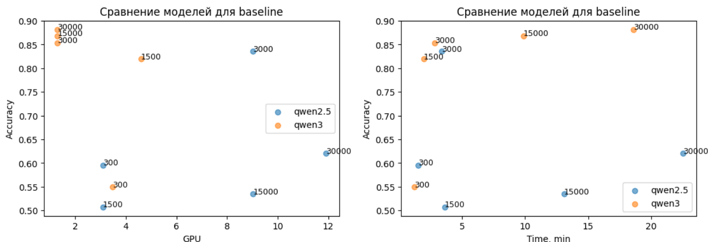
Заменить картинки на актуальные Рисунок 3. Сравнение моделей по качеству, застратам GPU и времени для baseline с указанием объема обучающей выборки
