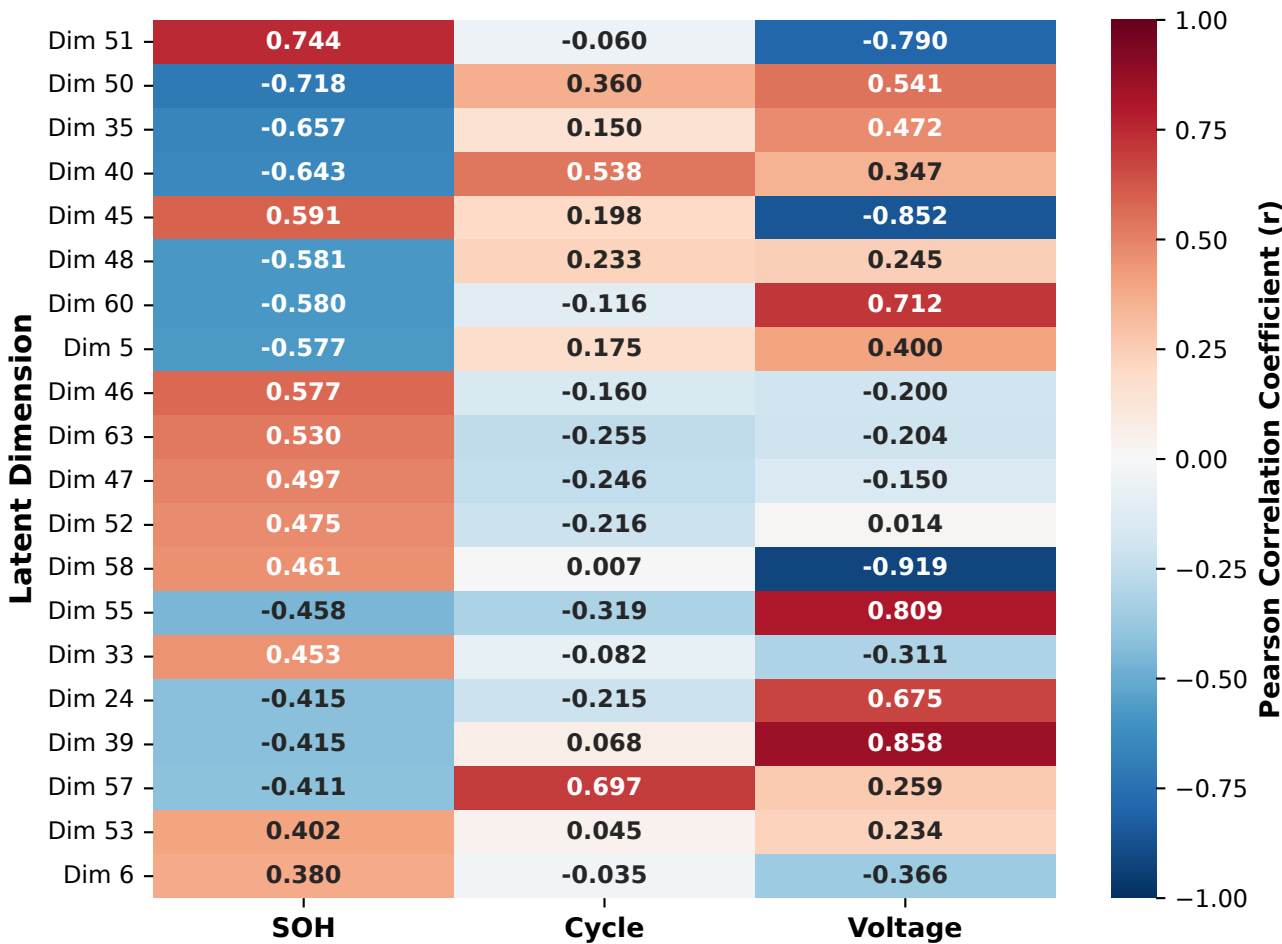
(d) CALB (CALB)
