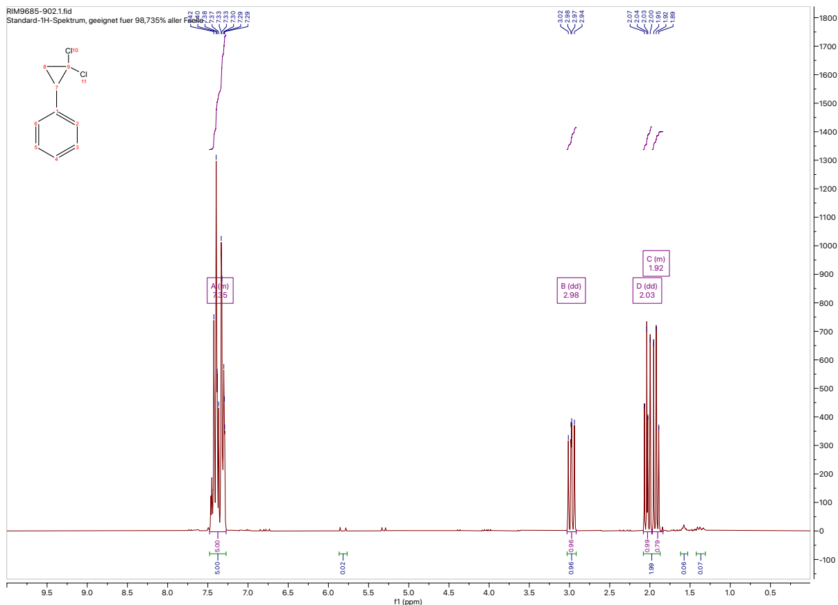
Abbildung 4: ^1\text{H} -NMR Spektrum des erhaltenen Produkts 1,1-Dichlor-2-phenylcyclopropan
