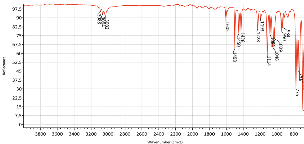
Abbildung 3: IR-Spektrum des Produkts 1,1-Dichlor-2-phenylcyclopropan
