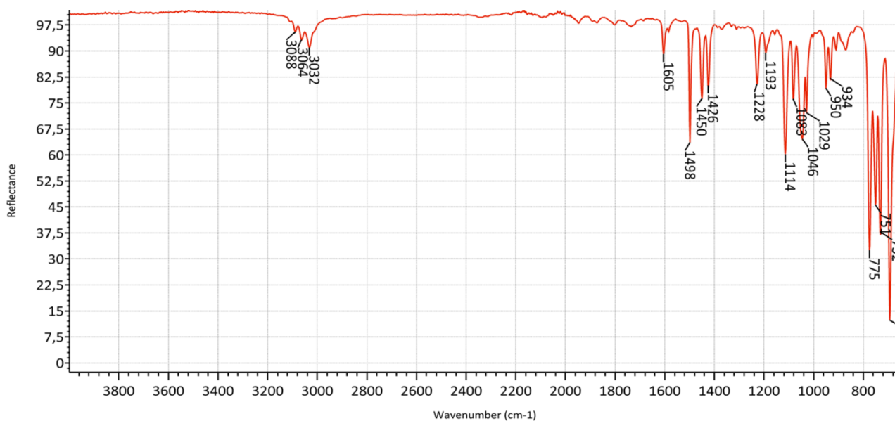
Abbildung 4: IR (1,1-Dichlor-2-phenylcyclopropan): \tilde{\nu} (cm -1 ) = 3088, 3064, 3032 (aromat. und aliph. C–H), 1605, 1498 (aromat. C = C), 775, 751, 732 (aromat. C–H und C–Cl).
