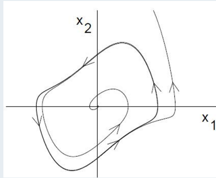
图 10: 极限环
