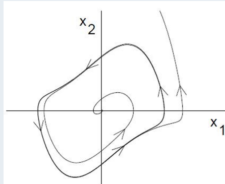
图 10: 极限环
