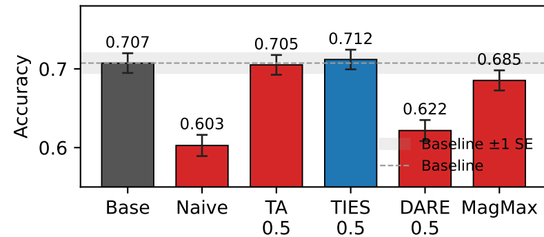
GSM8K
