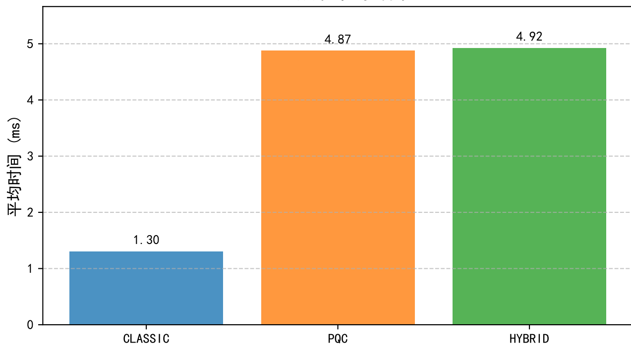
TLS握手平均时间
