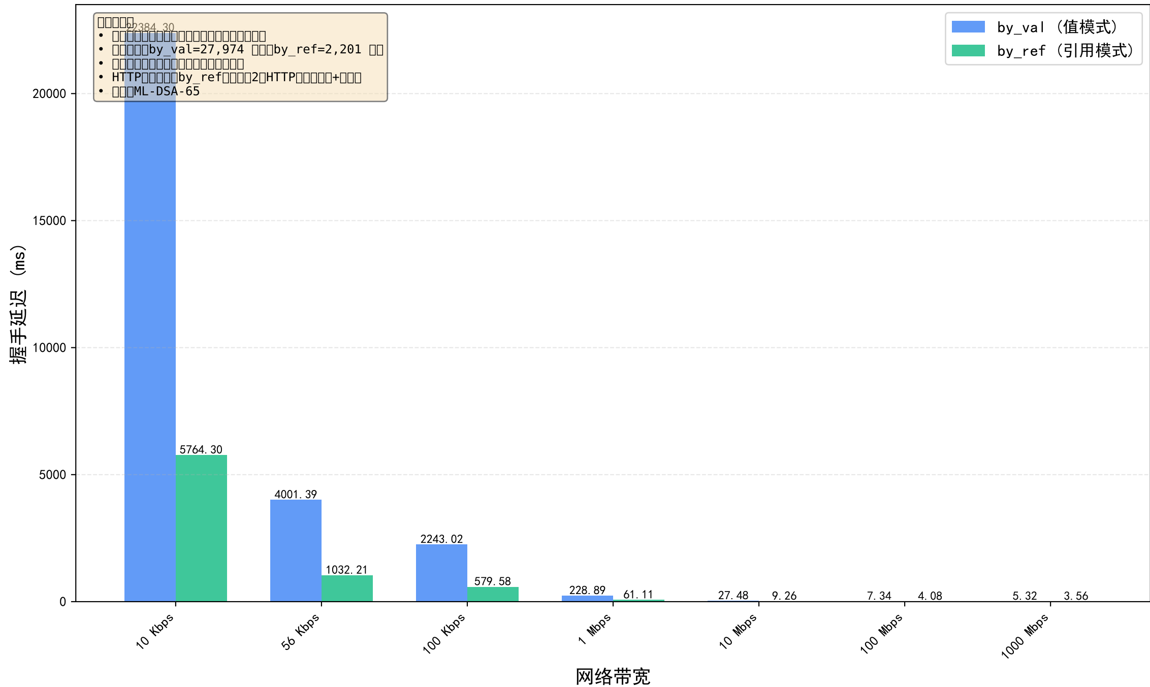
不同网络带宽下的握手延迟对比 (本地回环, ML-DSA-65算法)
