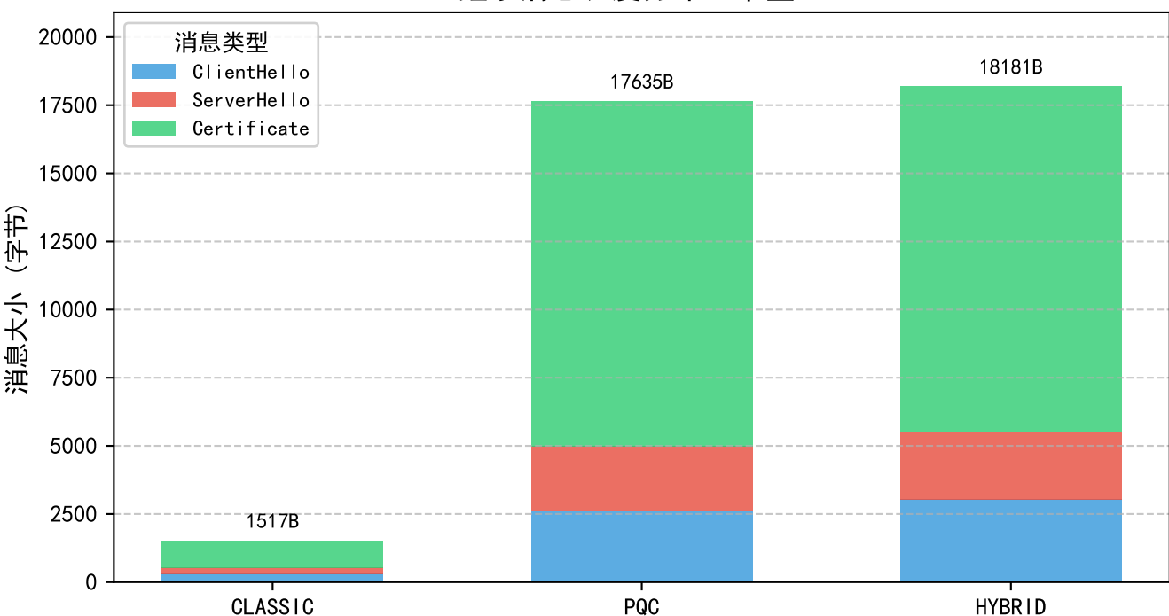
握手消息长度分布（堆叠）
