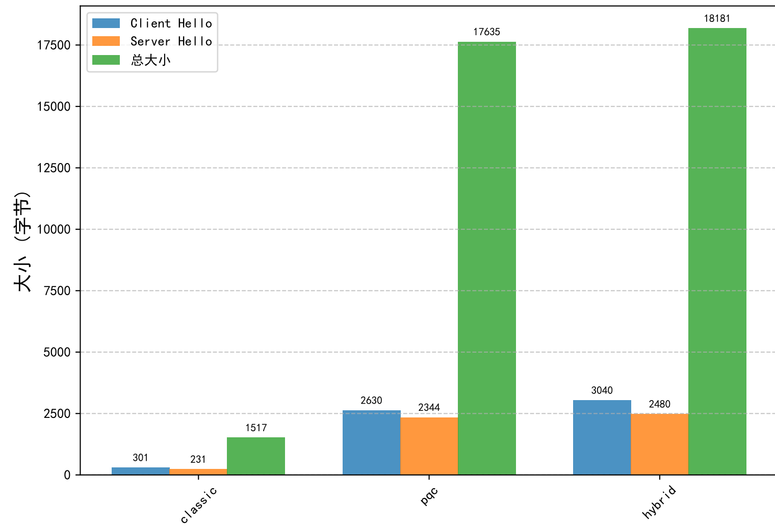
TLS握手消息大小比较
