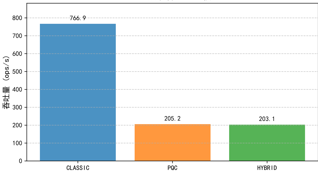
TLS握手吞吐量比较
