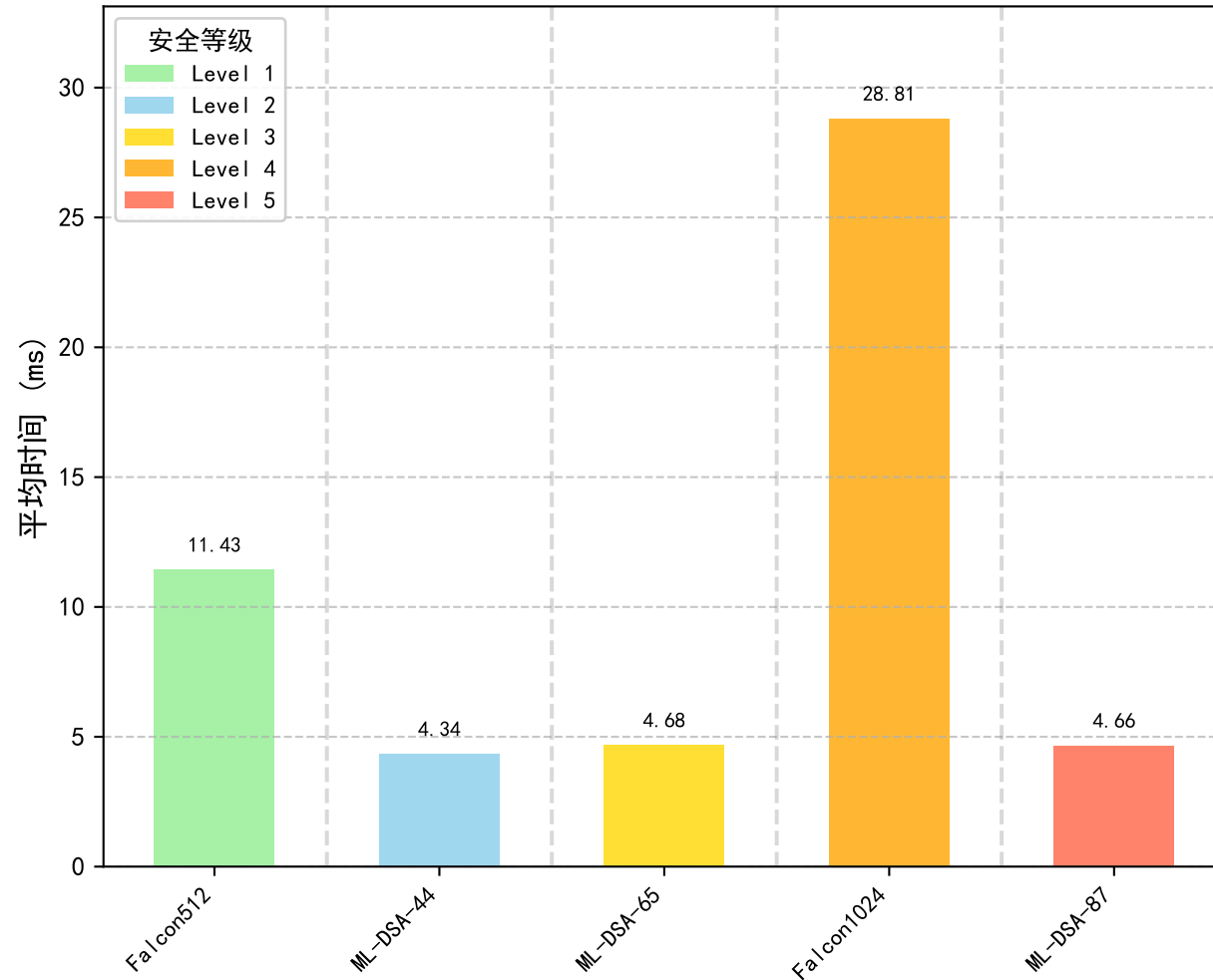
签名算法平均时间（按安全等级分组）
