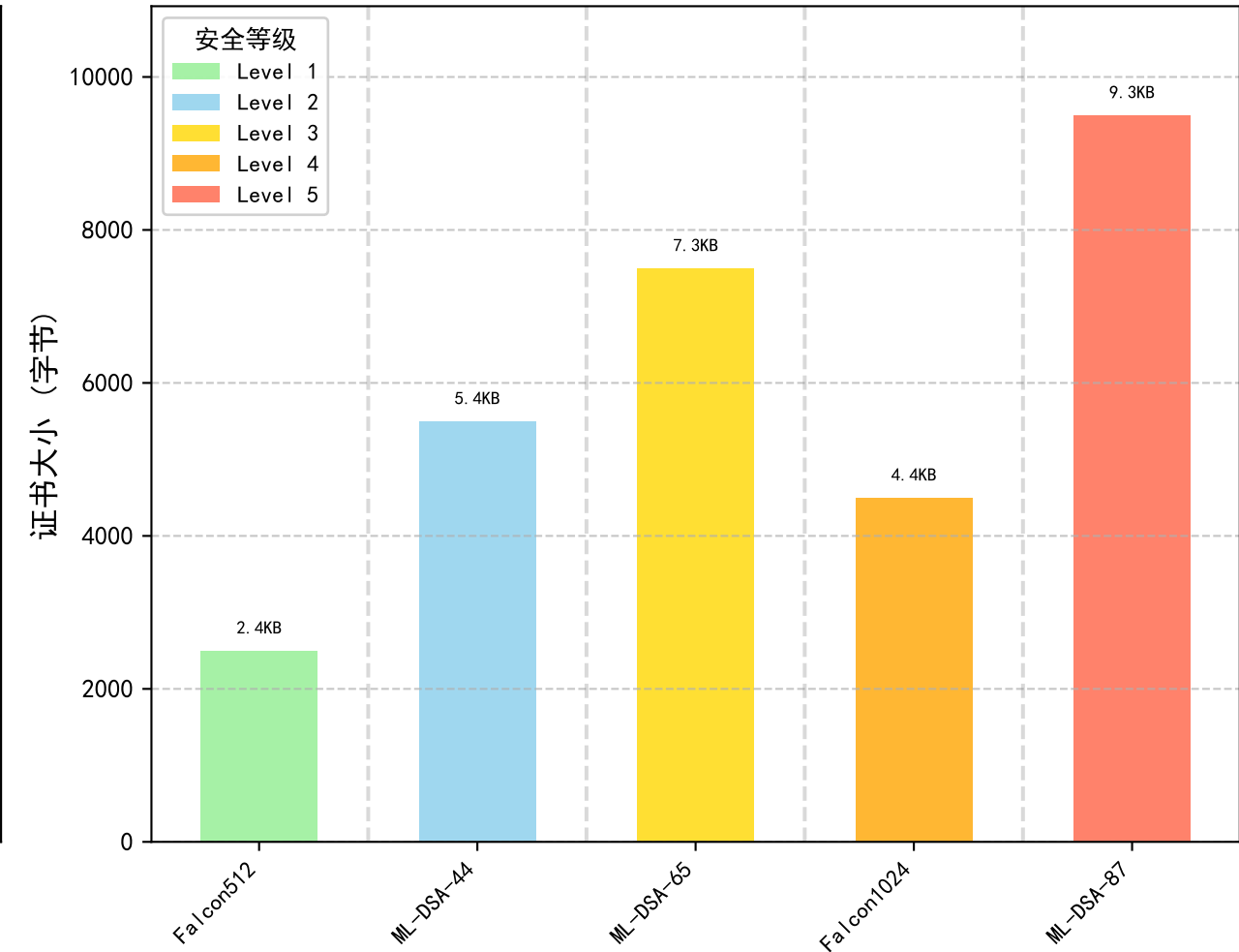
证书大小对比（按安全等级分组）
