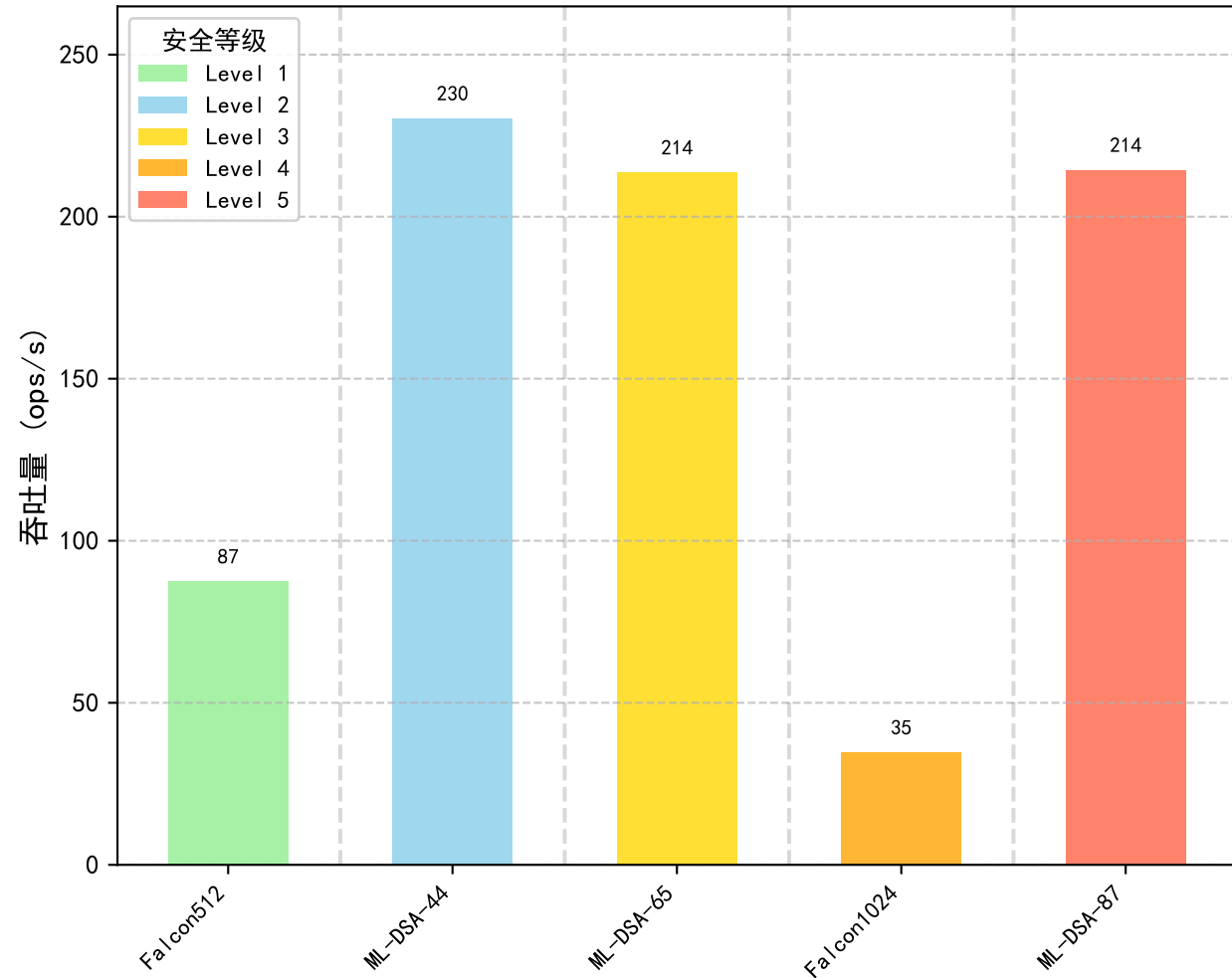
签名算法吞吐量比较（按安全等级分组）
