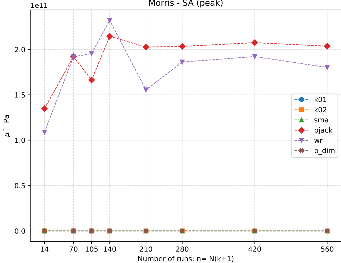
Morris - SA (peak)
