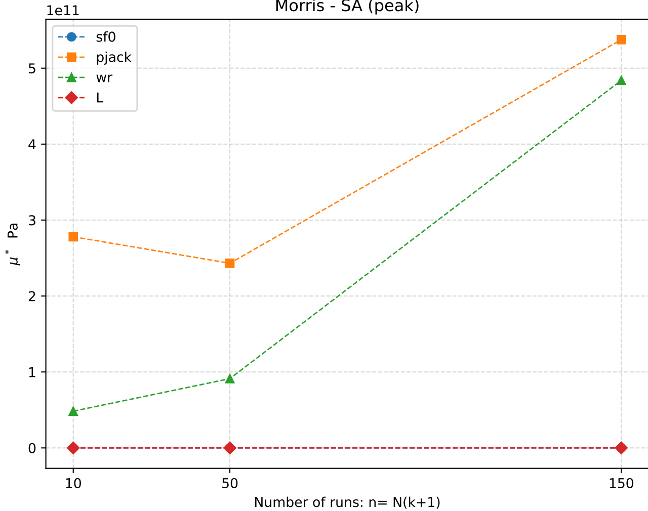
Morris - SA (peak)
