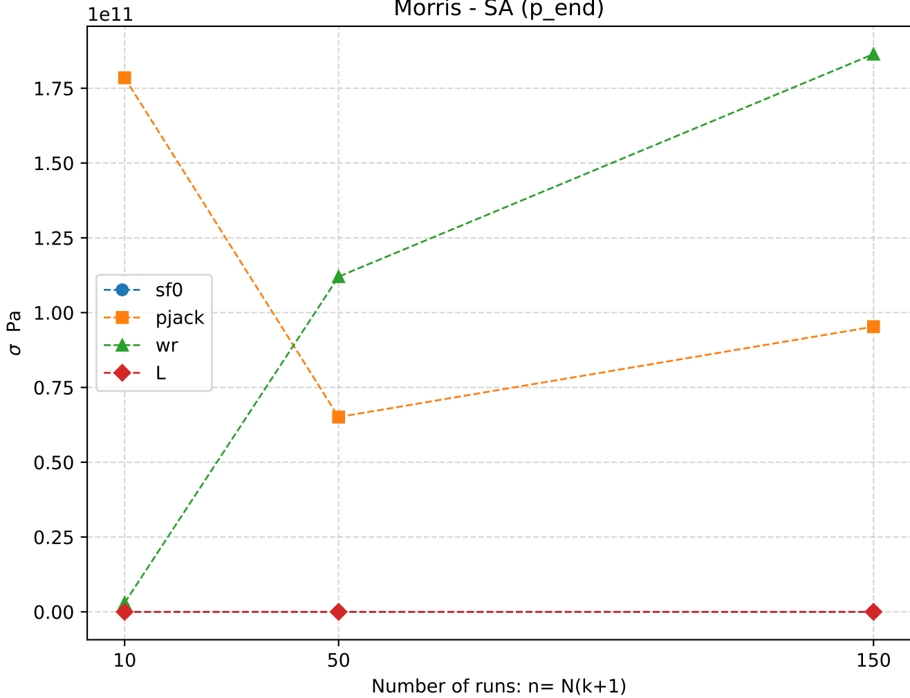
Morris - SA (p_end)
