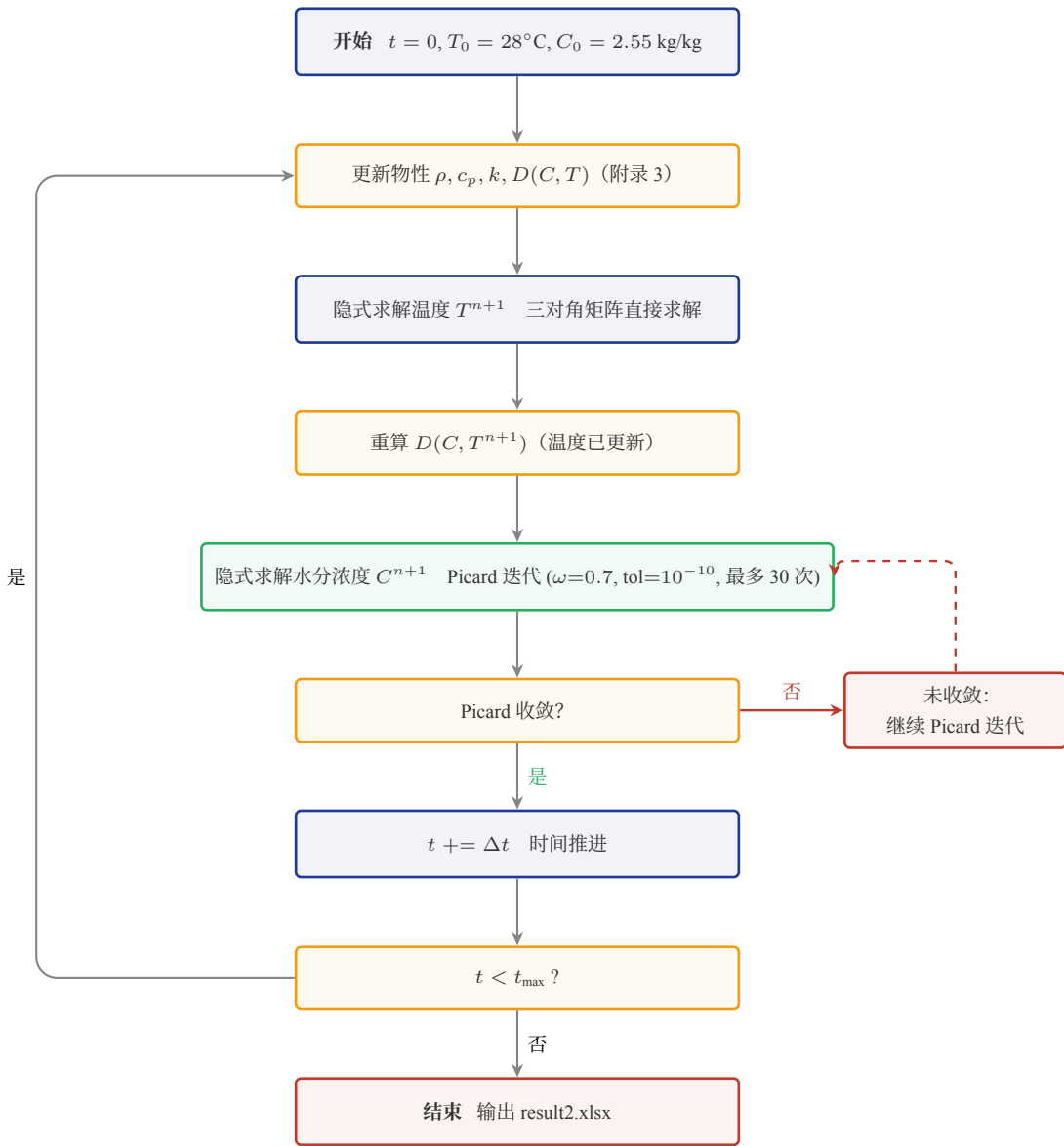
图 22：IMEX 交替推进算法流程
