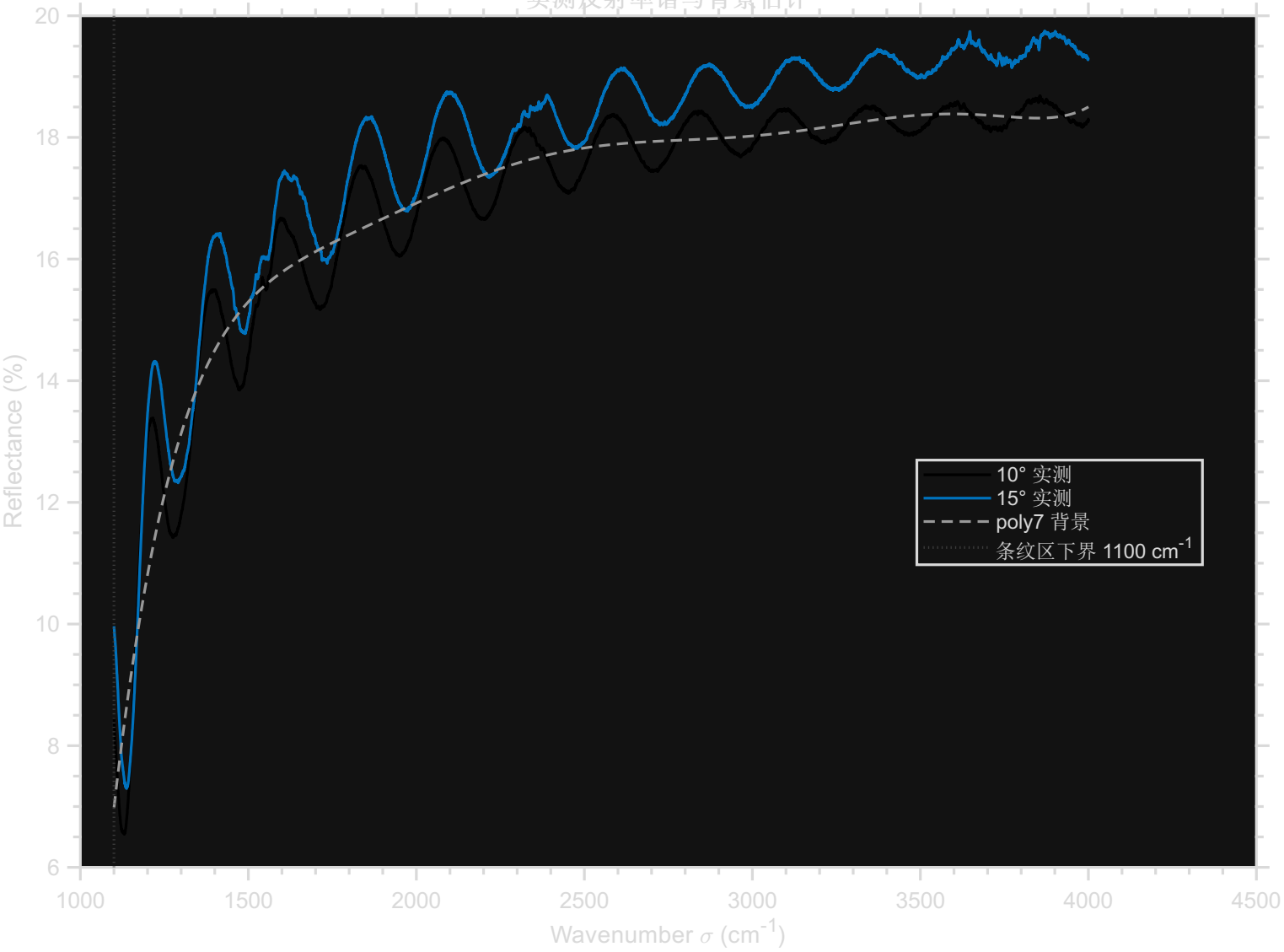
实测反射率谱与背景估计
