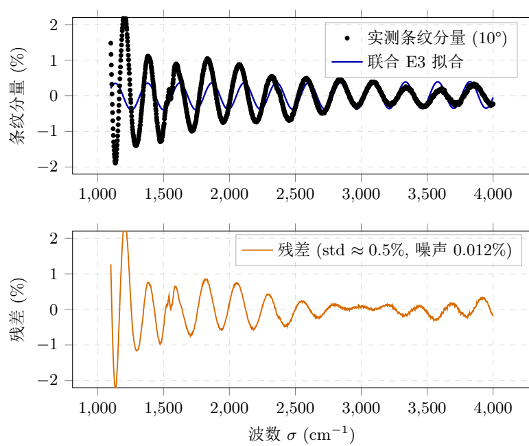
图 2: 联合 E3 拟合效果与残差 ( 10^\circ )。残差存在结构 (lag-1 自相关 0.999), 已归因并计入系统误差预算, 作为问题 3 模型升级的定量触发证据。
