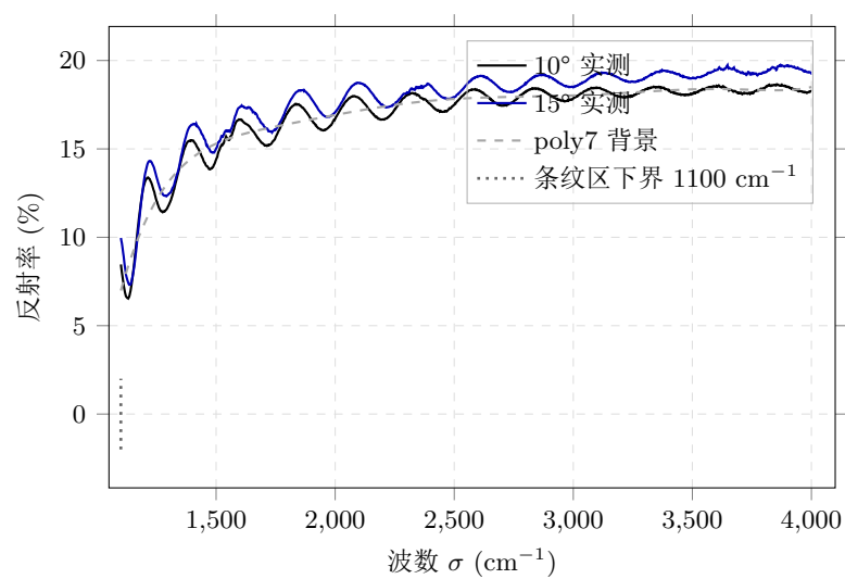
图 1: 实测反射率谱与背景估计 (10°/15°, 条纹区 \sigma \geq 1100 \text{ cm}^{-1} )
