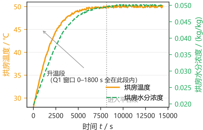
烘房环境条件时序
